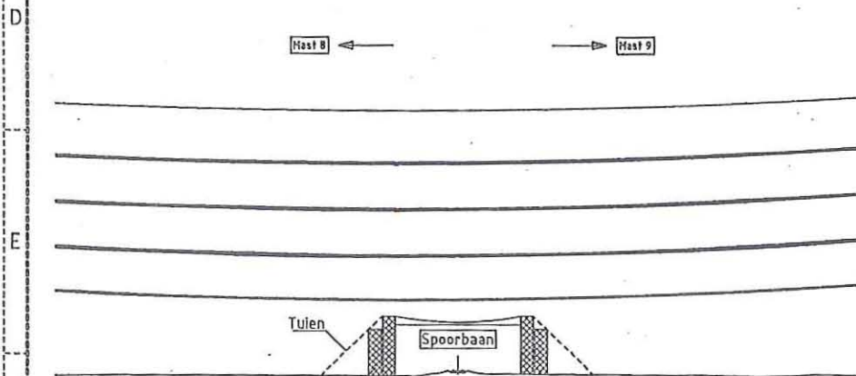
Doorsnede A-A
