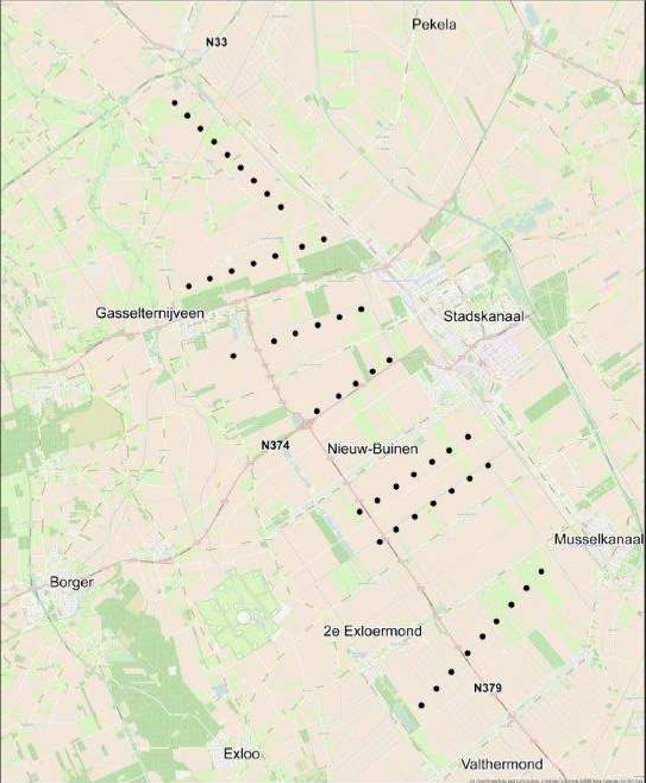
Indicatieve kaart van 150 MW verdeeld over 50 molens van 3MW in een opstelling van zeven lijnen
