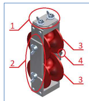
Figuur 3 Rollenstel
