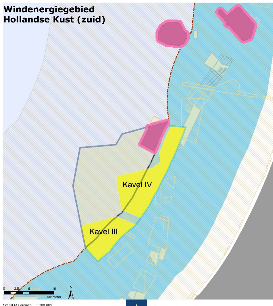
Figuur 3.2 Windenergiegebied Hollandse Kust (zuid) en (zand)wingebieden
