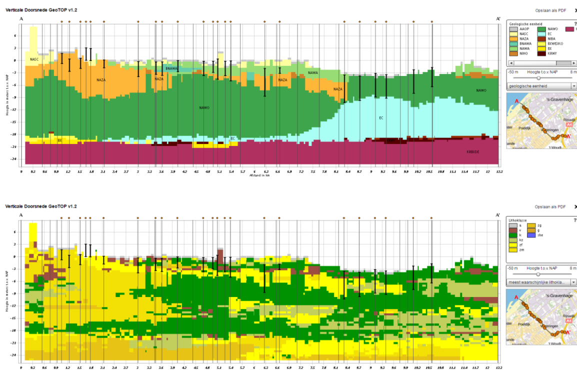
Afbeelding 4.5 Doorsnede GeoTOP v1.2 studiegebied nabij Wieringen. Boven: geologische eenheid. Onder: meest waarschijnlijke lithologische 1 klasse. (bruin is veen, groen is klei/kleig zand en geel is zand)
