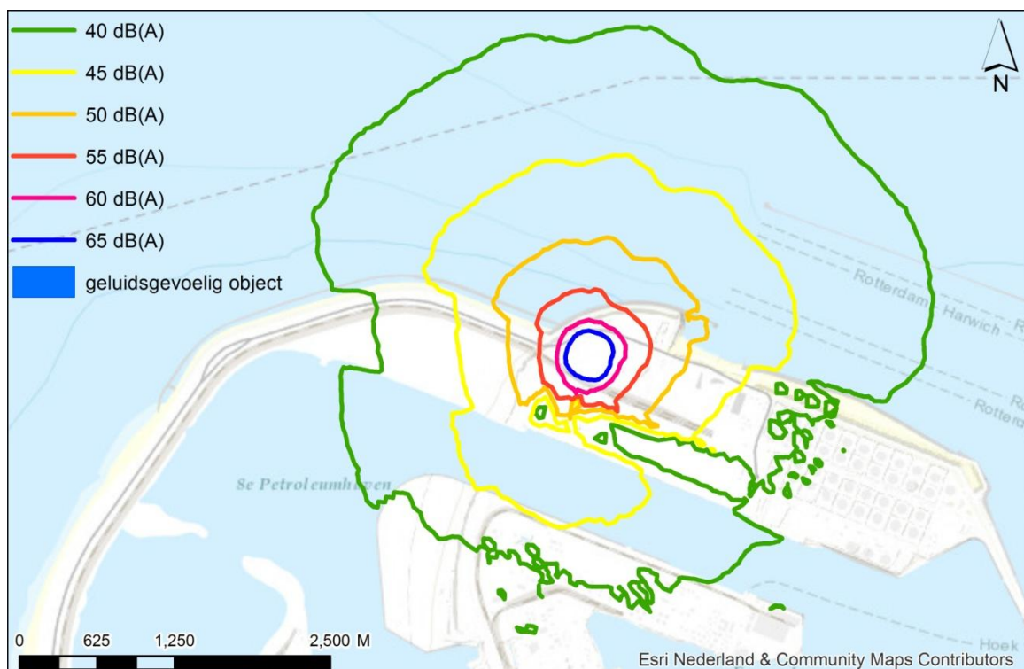
Afbeelding 8.9 Geluidcontouren gebruiksfase transformatorstation, voor mensen (van buitenaf is de derde contour 50 dB(A))
