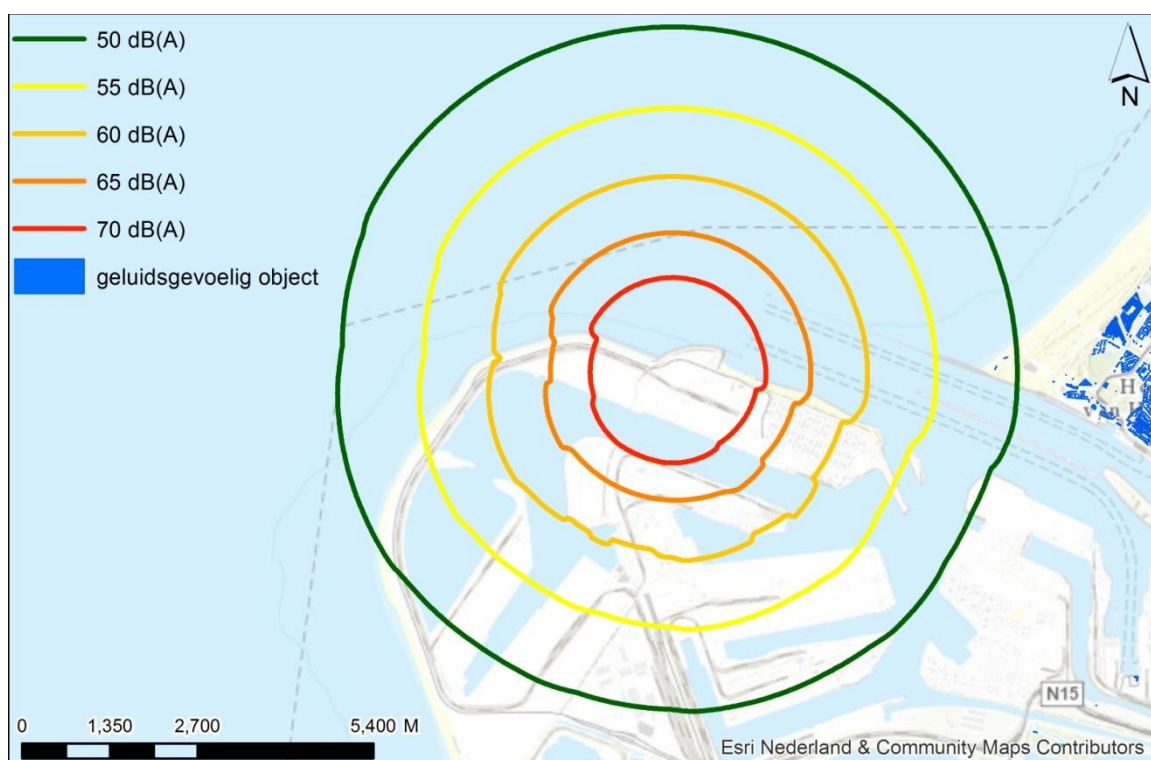
Afbeelding 8.5 Geluidcontouren aanlegfase transformatorstation, voor mensen
