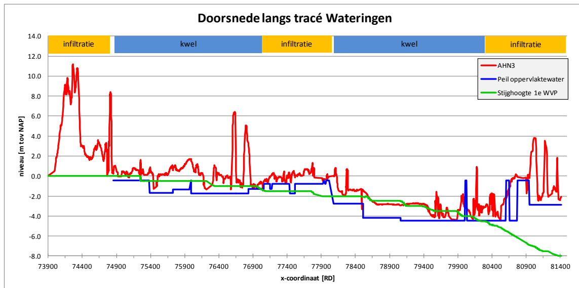
Afbeelding 4.3 Doorsnede grondwaterstand en stijghoogte langs tracé Wateringen
