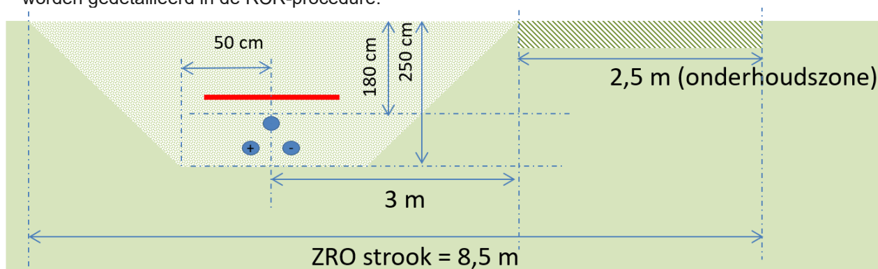
Figuur 2-5 Kabelbed op land bij een gelijkstroomverbinding
