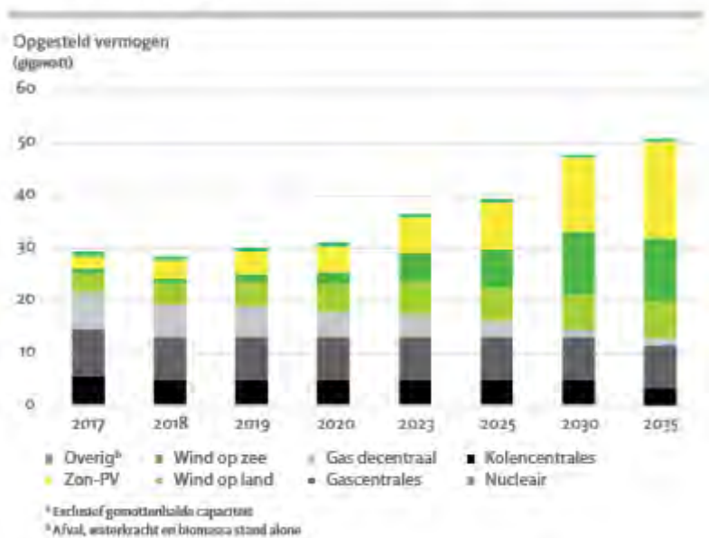
Figuur 4.2 Ontwikkeling opgesteld elektrisch vermogen in Nederland in de periode 2017-2035 1 .
