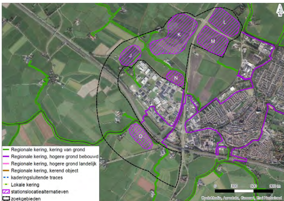
Afbeelding 8.5 Regionale waterkeringen in zoekgebied Bolsward
