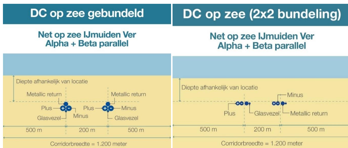
Figuur 2.2 Corridor gebundelde ligging kabeltracé op zee met paralleligging IJmuiden Ver Alpha en Beta Links: 1 bundel van 4 kabels. Rechts: 2 bundels van 2 kabels.
