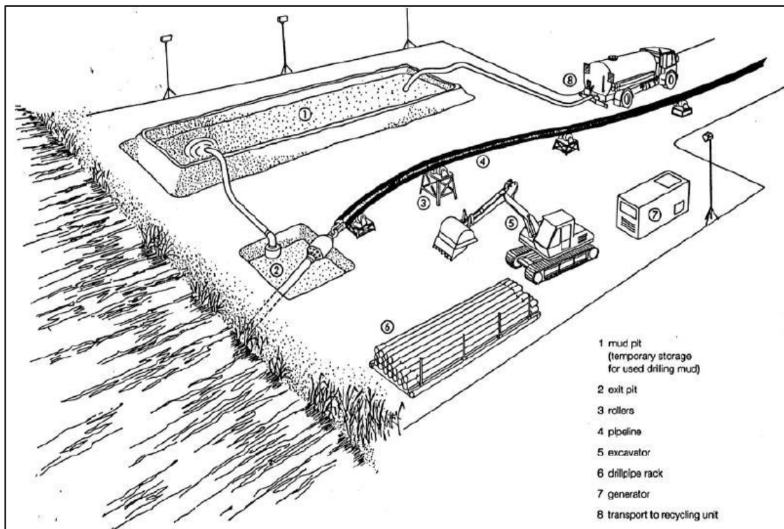
Figuur 2.9 Voorbeeld van de locatie bij en rondom een HDD intredepunt.
