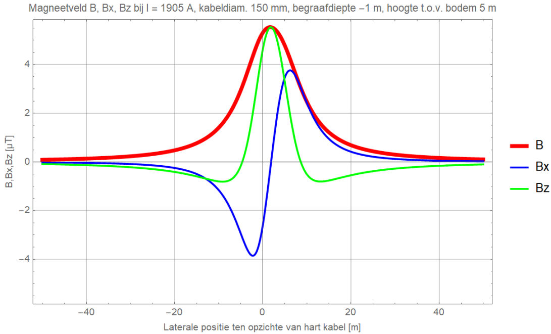
Figuur 8 (Onbalans / asymmetrie: DMR voert 10% retourstroom)
