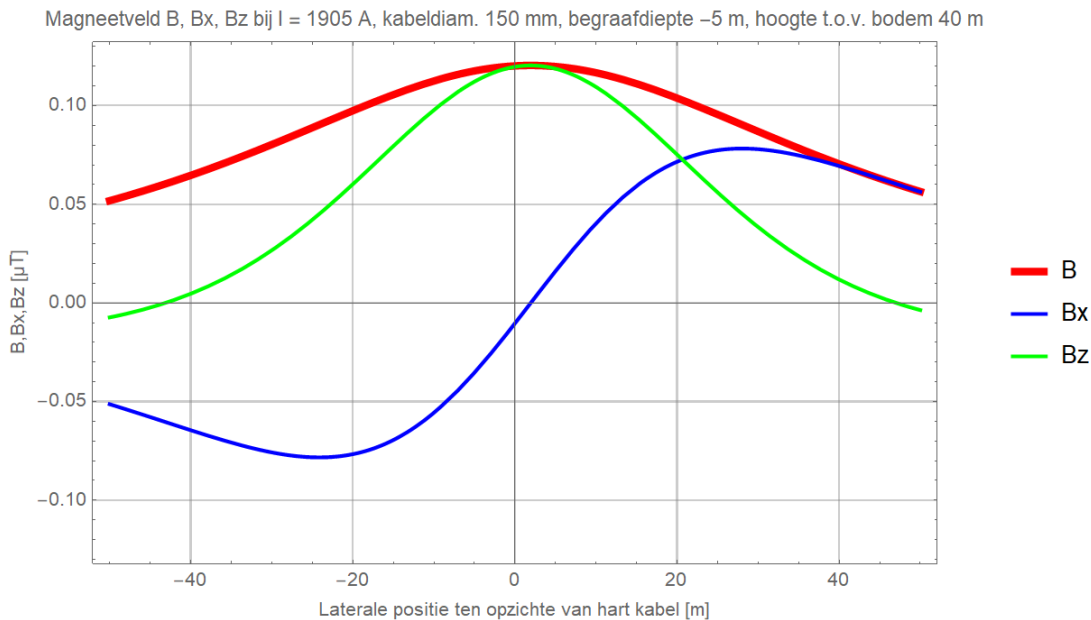
Figuur 37 (Onbalans / asymmetrie: DMR voert 10% retourstroom)
