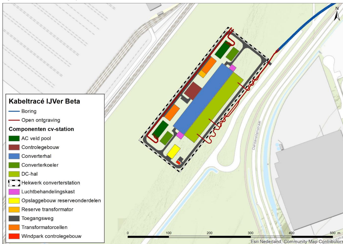
Figuur 2.11 Indicatieve lay-out van het converterstation
