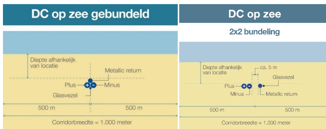
Figuur 2.1 Corridor gebundelde ligging kabeltracé op zee Links: 1 bundel van 4 kabels. Rechts: 2 bundels van 2 kabels.
