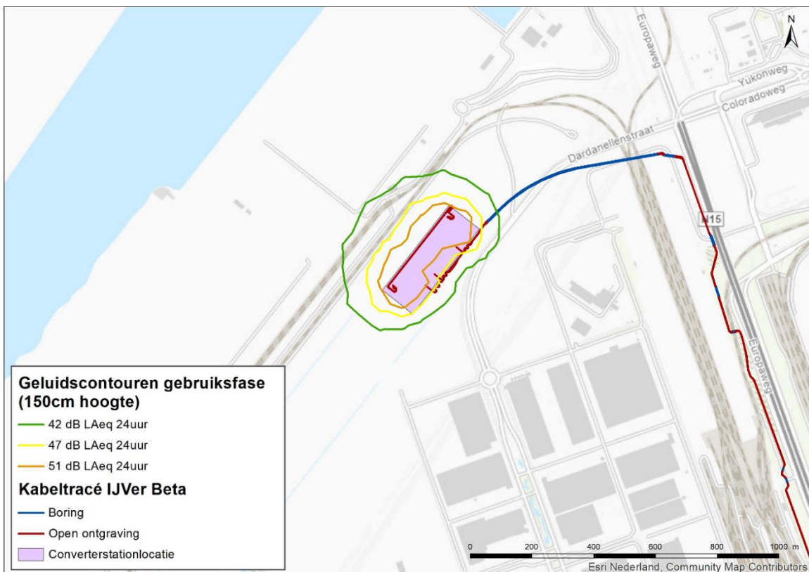
Figuur 34 Geluidscontouren 42 dB(A) 24eq in de gebruiksfase van het converterstation inclusief mitigerende, geluidsbeperekende maatregelen.
