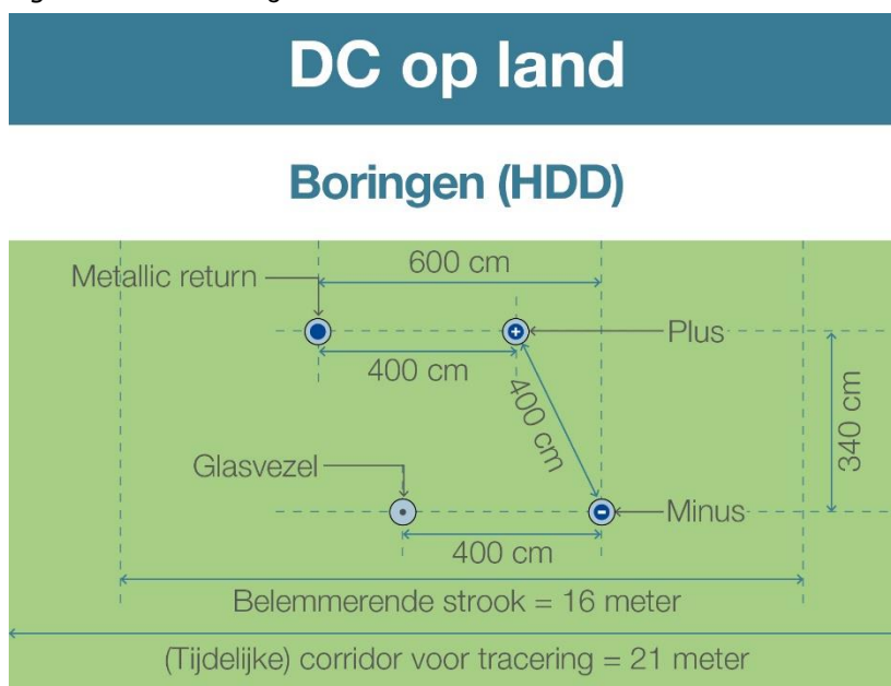
Figuur 2.7 HDD-configuratie voor DC 525kV-kabel.
