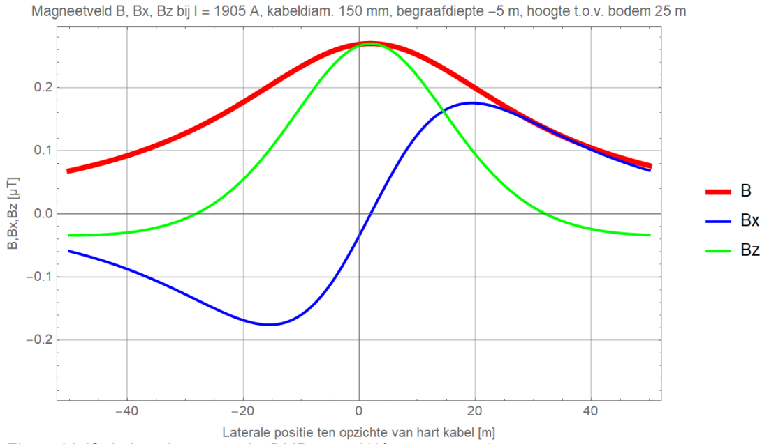
Figuur 36 (Onbalans / asymmetrie: DMR voert 10% retourstroom)
