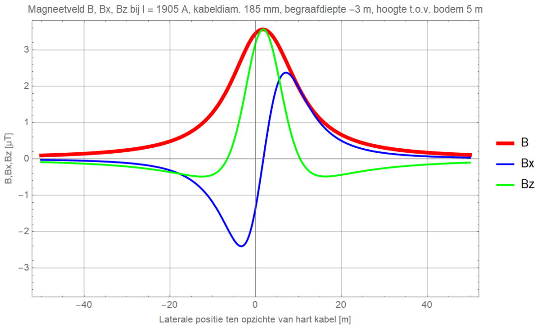
Figuur 56 (Onbalans / asymmetrie: DMR voert 10% retourstroom)
