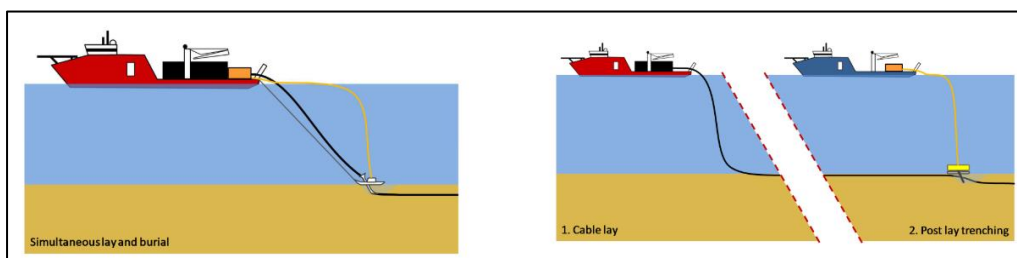
Figuur 2.3 Simultaneous Lay and Burial’ (links) en Post Lay Burial (rechts)
