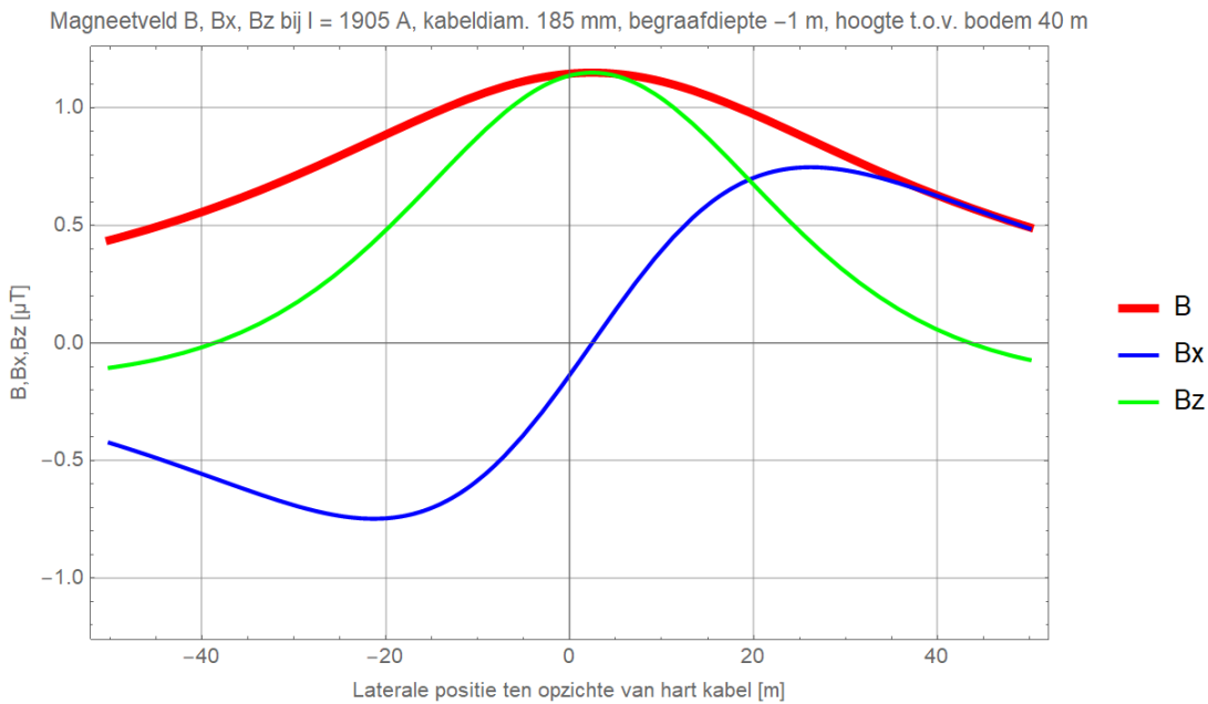
Figuur 109 (Storing / onderhoud, monopoolbedrijf: DMR voert 100% retourstroom)
