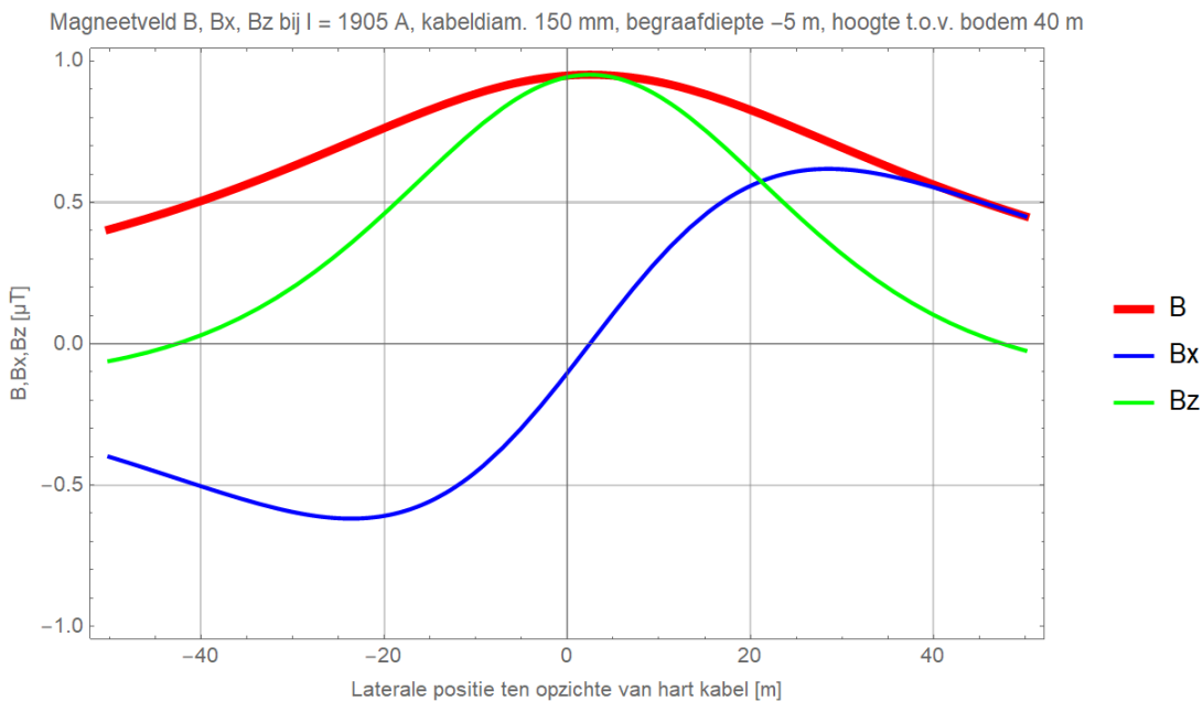
Figuur 101 (Storing / onderhoud, monopoolbedrijf: DMR voert 100% retourstroom)
