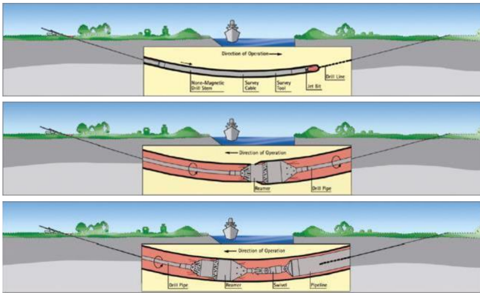
Figuur 2.8 De drie stappen van een horizontale boring.
