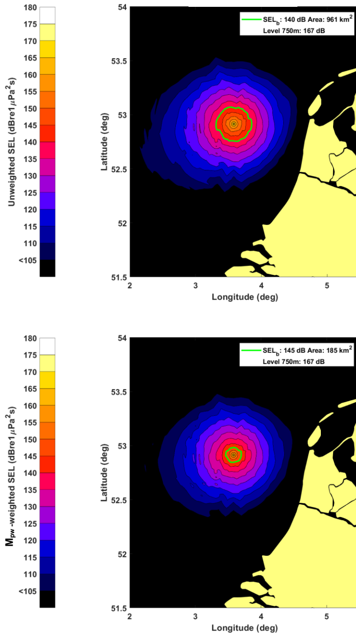
Figuur 2 Met Aquarius 4 berekende geluidskarten (SELs) en verstoringscontouren voor bruinvissen (boven) en zeehonden (onder) voor het heien van de fundering voor het Beta-platform voor de IJmuiden Ver windparken.
