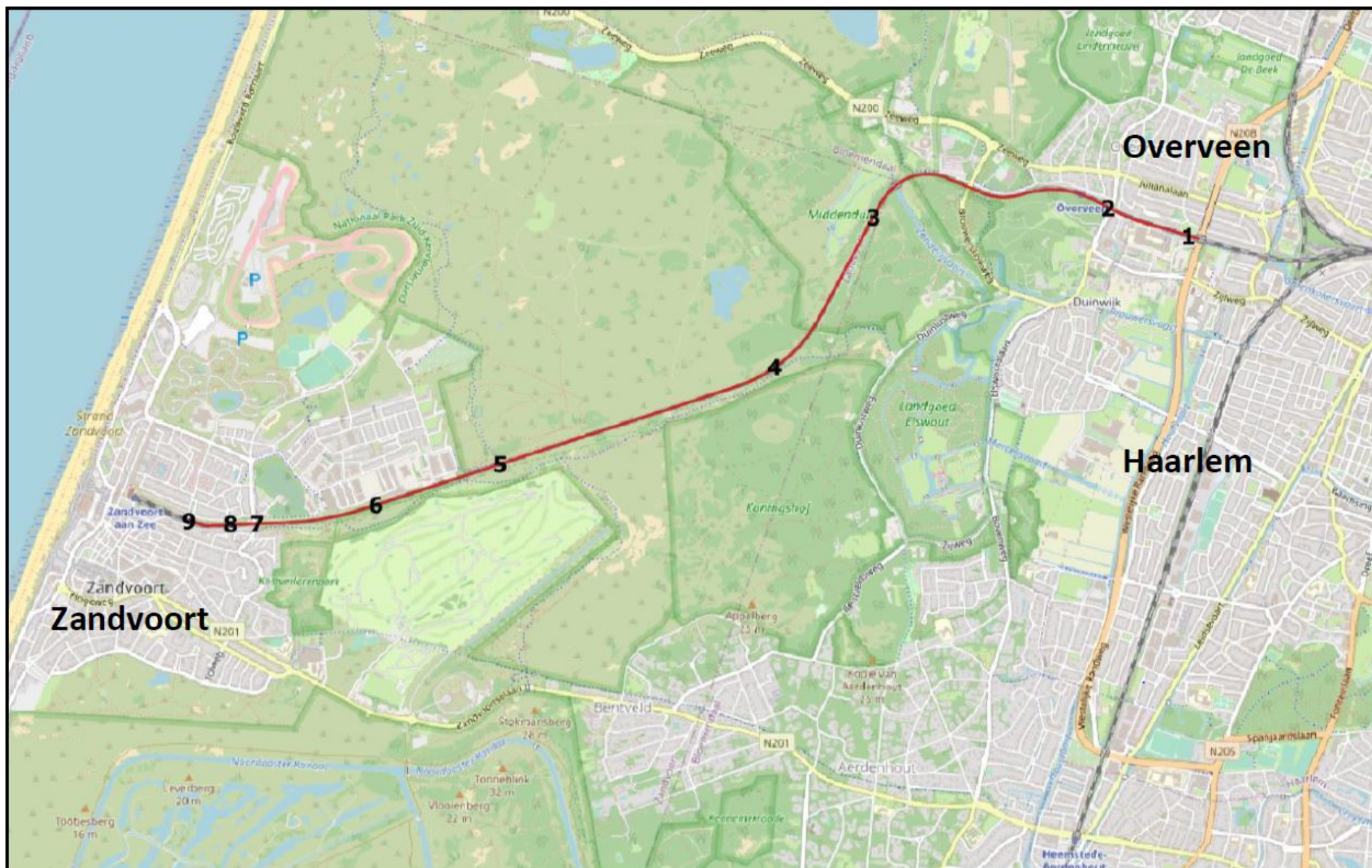
Figuur 1. Globale ligging van het projectgebied. De nummers indiceren de projectlocaties van 3kV voedingskasten. Nummers 3 (km 3.5 ) en 4 (km 4.5) betreffen de relevante kasten voor de ontheffingsaanvraag.
