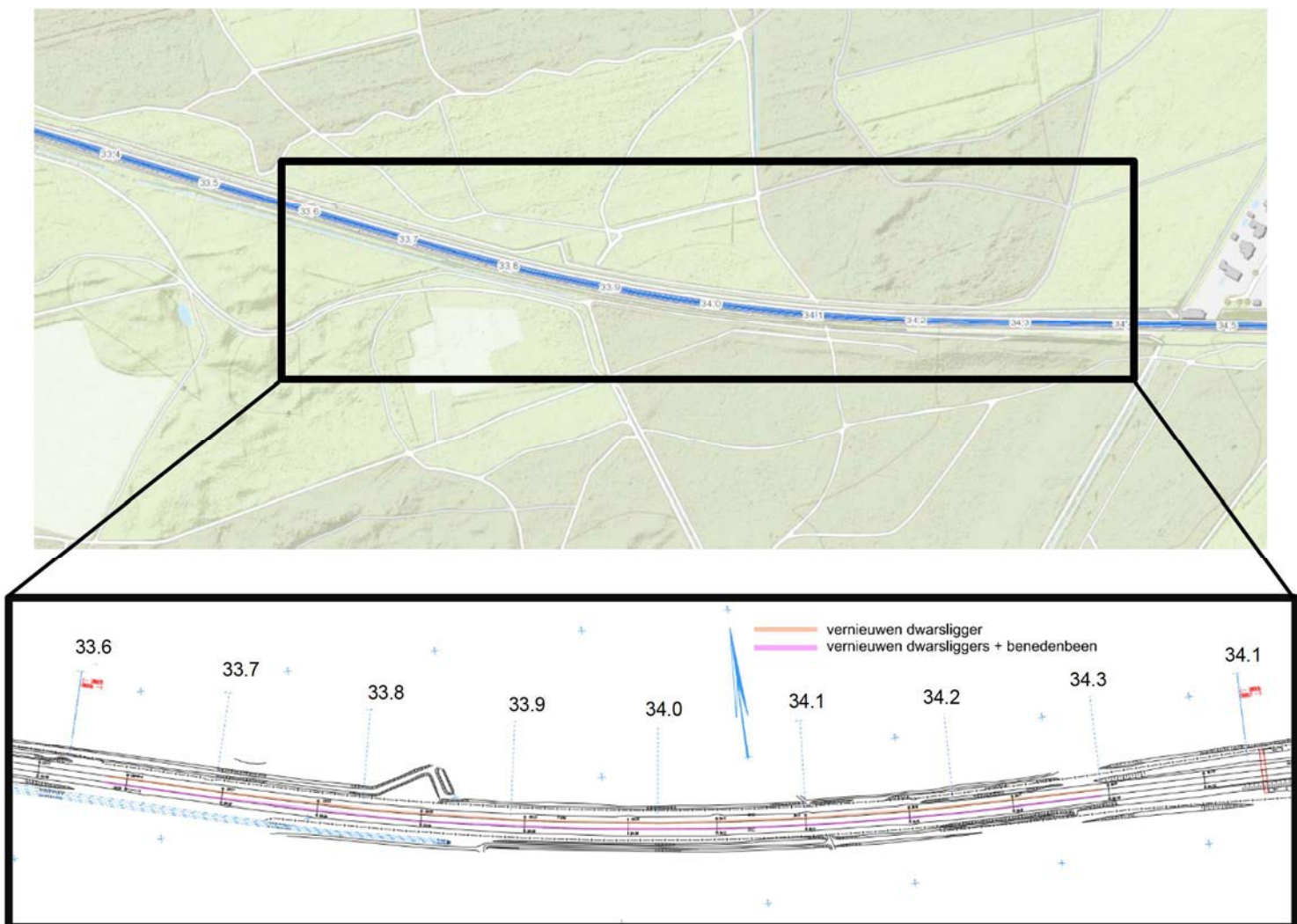
Figuur 2. Globale ligging van het traject met bijbehorende werkzaamheden waar een ontheffing voor wordt aangevraagd (BRON: BAMPRORAILGEODATA, 2022; ProjectspecificatiePRORAIL, 2021).
