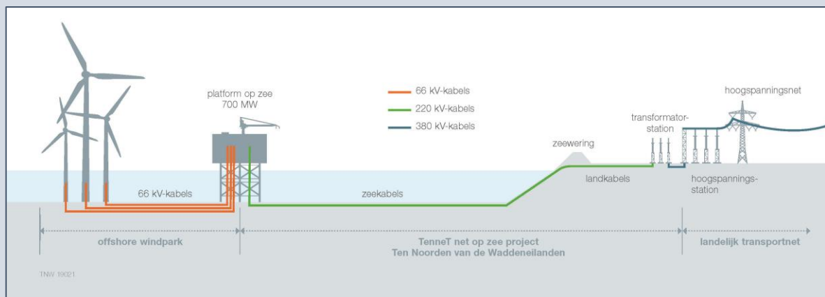
Afbeelding 4-1: Schematische weergave van benodigde infrastructuur op zee in het geval van wisselstroom
