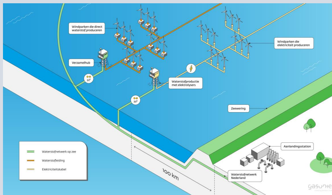
Afbeelding 4-10: Overzicht van aanlanding van waterstof
