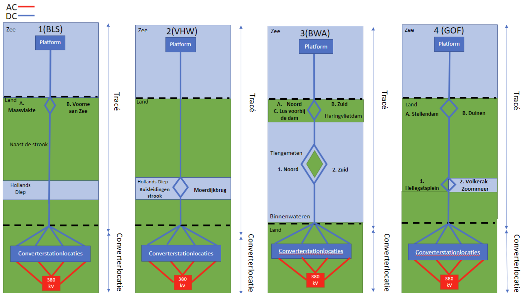
Figuur 3-9 Schematische weergave tracéalternatieven
