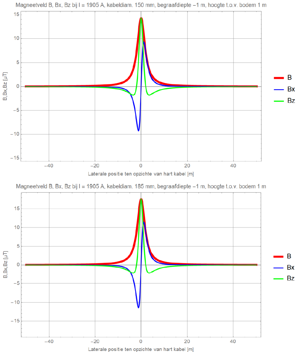
Figuur 4-6 Berekende magneetveldzone in \mu T van de 525kV-gelijkstroomkabels op zee bij een kabeldiameter van 150 mm (boven) en 185 mm (onder) voor (1x4) -kabelconfiguratie. Het magneetveld B is opgebouwd uit een horizontale en verticale component (Bx en Bz). Alleen het gehele magneetveld (B) zal van toepassing zijn. De (2x2)-kabelconfiguratie is vergelijkbaar met deze berekeningen. Afkomstig van van Essen (van Essen, 2020).
