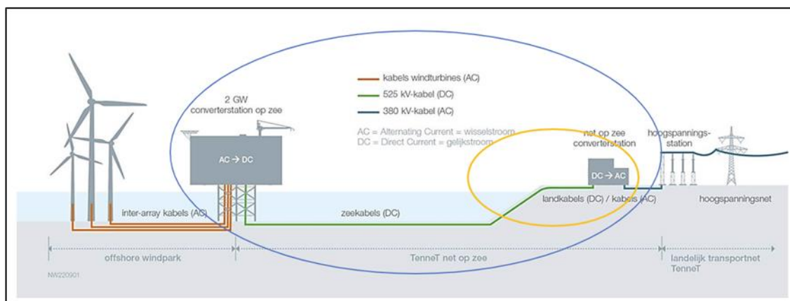
Figuur 1-1 Onderdelen van het voornemen Net op zee Nederwiek 3. Gele cirkel onderdelen MER fase 1 en blauwe cirkel onderdelen MER fase 2
