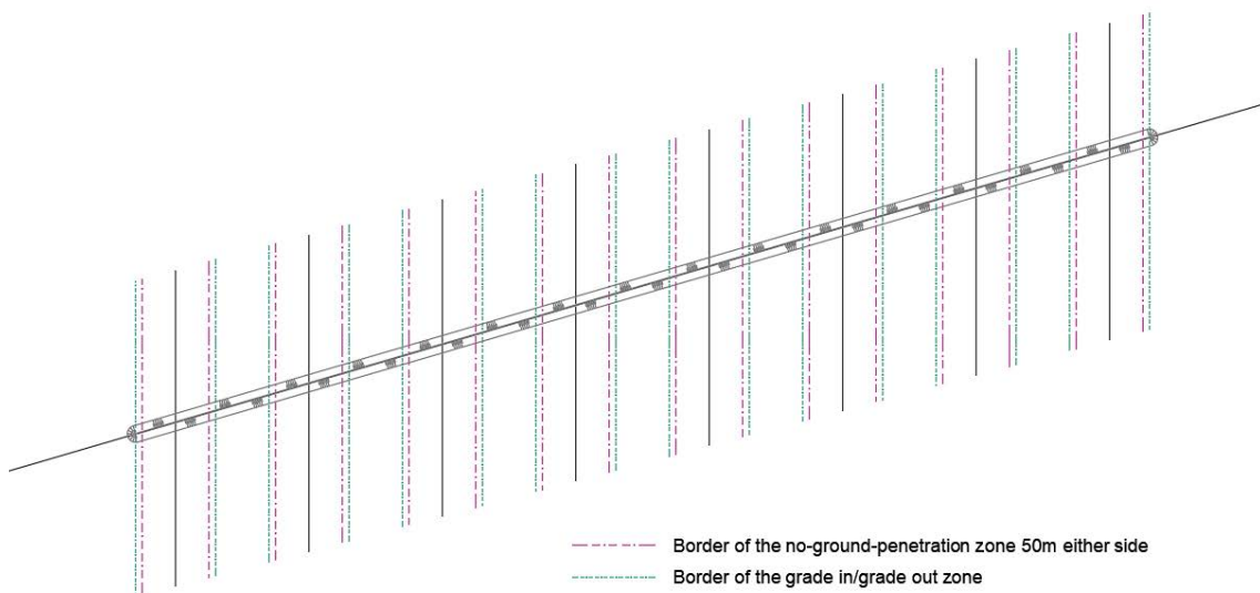
Figuur 4-6 Kruisingsbouwwerk voor acht kruisingen door middel van één continue steenberg
