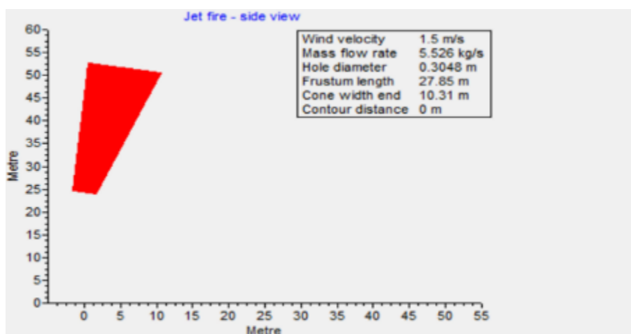
Figuur 5.18. Berekening vlamhoogte affakkelen productielocatie zij aanzicht (bron: MER Gaswinning en gasboring Ternaard)
