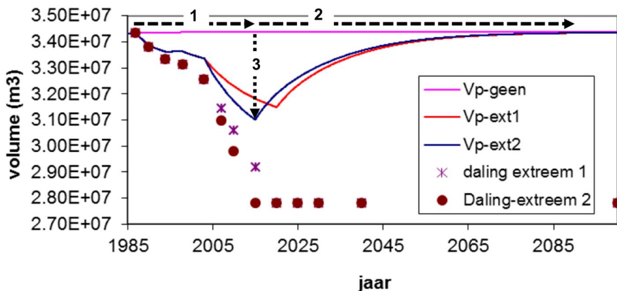
Figuur 8-1 Grafiek met de ontwikkeling van het bodemdalingsvolume in het Pinkegat bij twee scenario's 'extreem 1' en 'extreem 2' (de punten in de grafiek), de ontwikkeling van het volume sediment in de droogvallende plaat (Vp-geen), en de ontwikkeling van het sedimentvolume in de plaat onder invloed van de twee bodemdalingsscenario's (Vp-ext1: extreem 1 en Vp-ext2: extreem 2). Afkomstig uit Wang et al. (2017)
