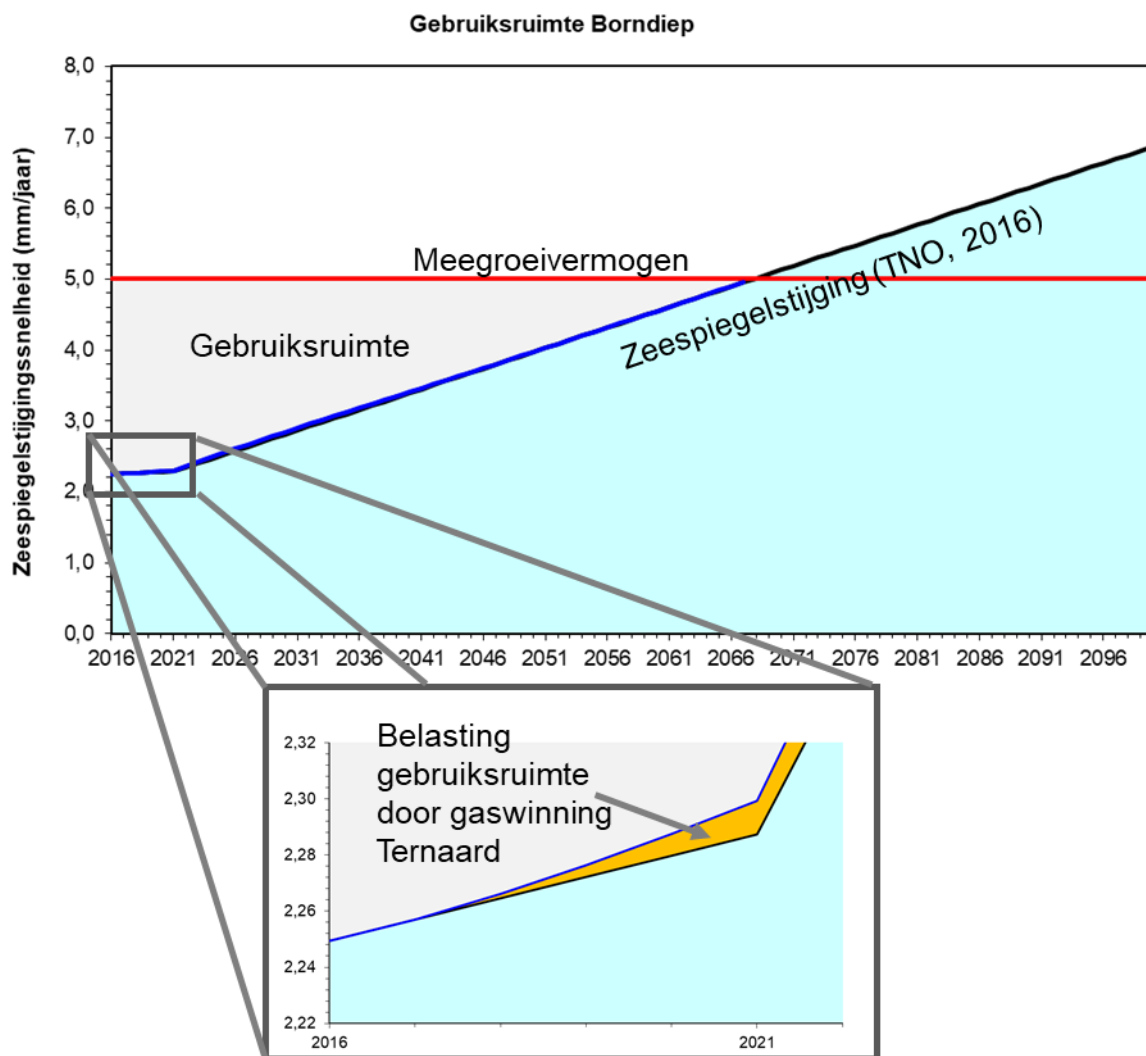
Figuur 4-2 Grafiek met de voorspelde belasting van de gebruiksruijtte voor de Voorgenomen gaswinning Ternaard (de blauwe lijn) voor het kombergingsgebied Borndiep. De rode lijn is de natuurgrens van 5 mm/jaar voor het Borndiep. De bovengrens van het lichtblauw gekleurde vlak geeft het zeespiegelstijgingsscenario TNO 2016. Het grijze vlak is de nog beschikbare gebruiksruijtte
