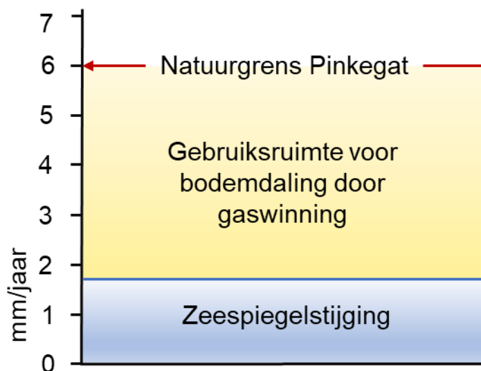
Figuur 3-8 Schematische weergave van de relaties tussen de natuurgrens als maat voor het meegroeivermogen van een kombergingsgebied, de zeespiegelstijging en de gebruiksruimte voor gaswinning onder dat kombergingsgebied. De snelheid van zeespiegelstijging in deze figuur is de huidige waargenomen snelheid, ontleend aan Baart et al 2018)
