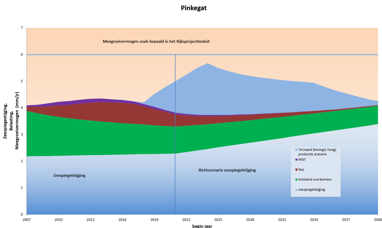
Figuur 4-1 Grafiek met de voorspelde belasting Ternaard bij de voorgenomen gaswinning binnen de gebruikruimte voor de Ternaard bodemdaling en de bestaande gaswinning Ameland en MLV (Nes, MGT) voor het kombergingsgebied Pinkegat (zeespiegelstijgingsscenario TNO 2016)
