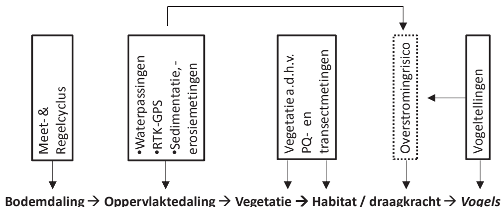
Figuur 7: Effectketen kwelder (vet gedrukt) en de daaraan gekoppelde monitoringonderdelen (in de kaders). Het gestippelde kader "overstromingsrisico" wordt berekend uit de metingen voor oppervlakedaling en niet apart gemeten. De pijlen geven de koppeling tussen de onderdelen weer. De schakels "Habitat / draagkracht" vormen de instandhoudingsdoelen.
