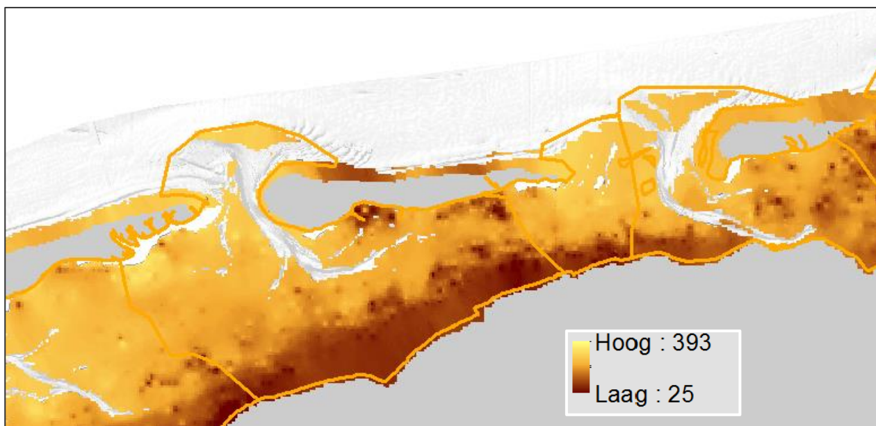
Figuur 7-4 Uitsnede uit de kaart van de mediane korrelgrootte (diameter in \mu\text{m} ) op basis van de SIBES-bemonstering (uit Christianen et al, 2015)
