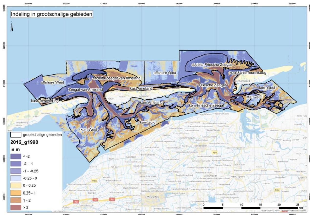
Figuur 7-2 Gebiedsindeling zoals gehanteerd voor de volumebepalingen door Vermaas en Marges (2015), op de vershilkaart 1990-2012 (uit Vermaas en Marges, 2015)
