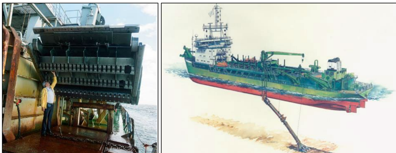
Figuur 3-4 Links: Foto van de sleepkop van een sleephopperzuiger (bron: beeldbank RWS). Rechts: Zijaanzicht van een sleephopperzuiger in werking met neergelaten sleepkop (bron: edugis.nl).
