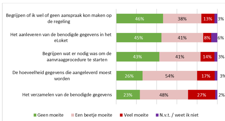
Figuur 4.8 Ervaren moeite met algemene aspecten van de aanvraagprocedure
