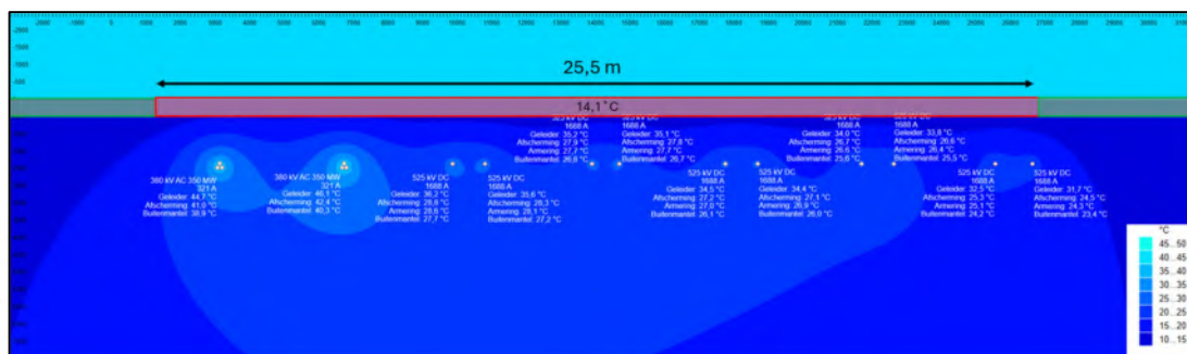
Figuur 14 - Grondtemperatuurontwikkeling kabelcorridor DRS0003 voor 10,7 GW scenario. Het rekenmodel voor de DC kabels is aangepast zodanig dat de juiste stroom door de polen gaat. Hierdoor geeft het figuur een waarde van 1688A neer, wat overeenkomt met de 975A zoals gegeven als uitgangspunt.
