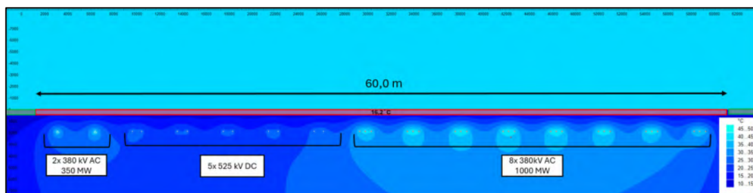
Figuur 16 – Grondtemperatuurontwikkeling kabelcorridor DRS0004 voor 10,7 GW scenario. Het rekenmodel voor de DC kabels is aangepast zodanig dat de juiste stroom door de polen gaat. Hierdoor geeft het figuur een waarde van 1688A neer, wat overeenkomt met de 975A zoals gegeven als uitgangspunt.
