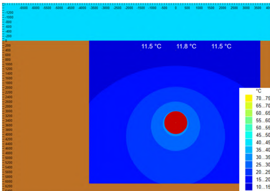
Figuur 17. Bodemtemperatuurprofiel voor één DN1200 waterstofleiding.
