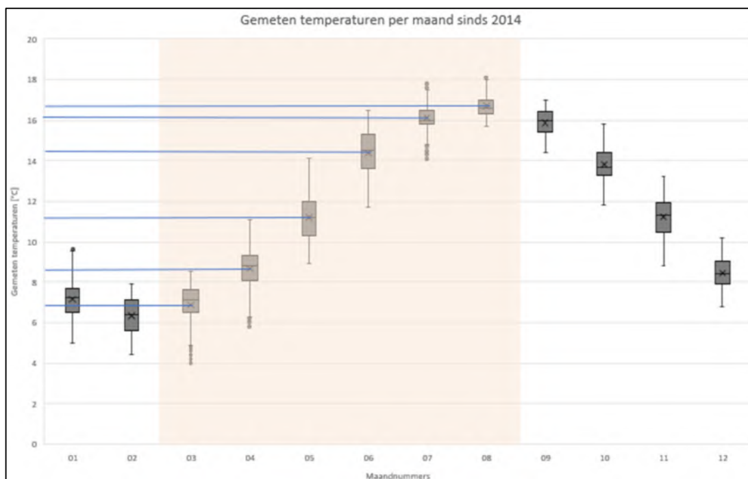
Figuur 3. Bodemtemperaturen op 0,5 meter diepte gemeten in Nieuw Beerta, Groningen sinds 2014.
