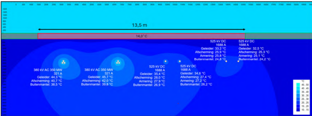
Figuur 13 - Grondtemperatuurontwikkeling kabelcorridor DR50003 voor 4,7 GW scenario. Het rekenmodel voor de DC kabels is aangepast zodanig dat de juiste stroom door de poleen gaat. Hierdoor geeft het figuur een waarde van 1688A neer, wat overeenkomt met de 975A zoals gegeven als uitgangspunt.
