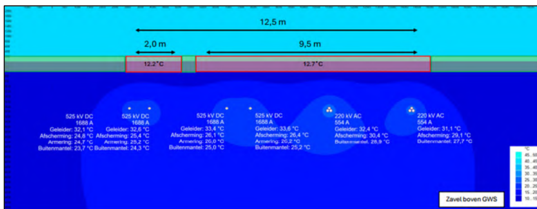
Figuur 11 - Grondtemperatuurontwikkeling kabelcorridor DRS0001 voor 4,7 GW scenario. Het rekenmodel voor de DC kabels is aangepast zodanig dat de juiste stroom door de polen gaat. Hierdoor geeft het figuur een waarde van 1688A neer, wat overeenkomt met de 975A zoals gegeven als uitgangspunt.
