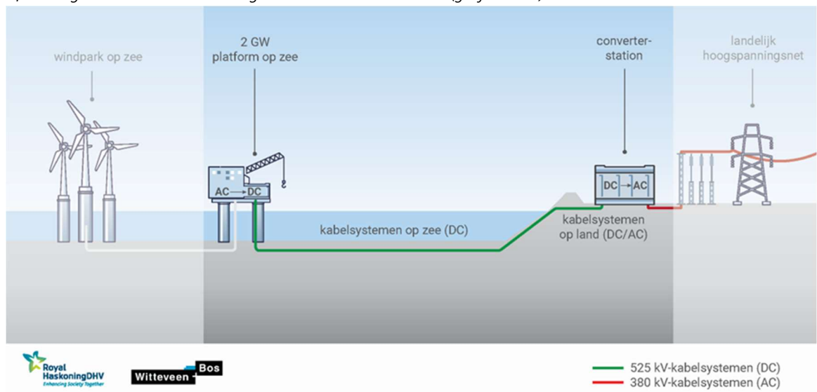
Afbeelding 1.2 - Schematische weergave van het elektriciteitsnet (gelijkstroom).
