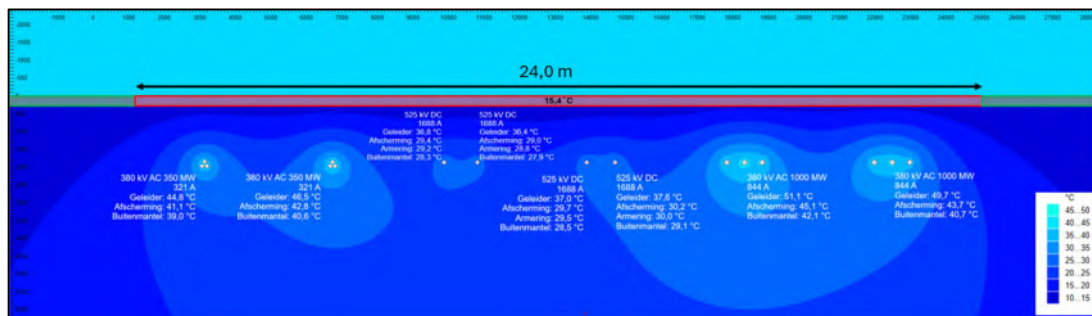
Figuur 15 - Grondtemperatuurontwikkeling kabelcorridor DRS0004 voor 4,7 GW scenario. Het rekenmodel voor de DC kabels is aangepast zodanig dat de juiste stroom door de polen gaat. Hierdoor geeft het figuur een waarde van 1688A neer, wat overeenkomt met de 975A zoals gegeven als uitgangspunt.
