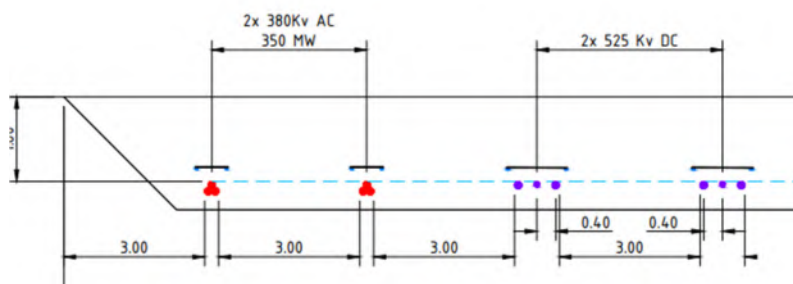
Figuur 7 - Kabelcorridor cross section 3 voor 4,7 GW scenario.
