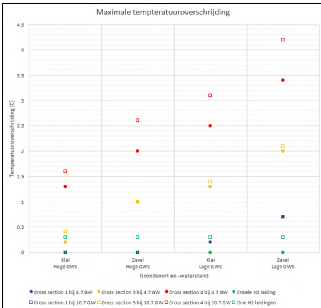
Figuur 19. Maximale temperatuuroverschrijdingen t.o.v. grondslagen en -waterstanden voor de verschillende configuraties.
