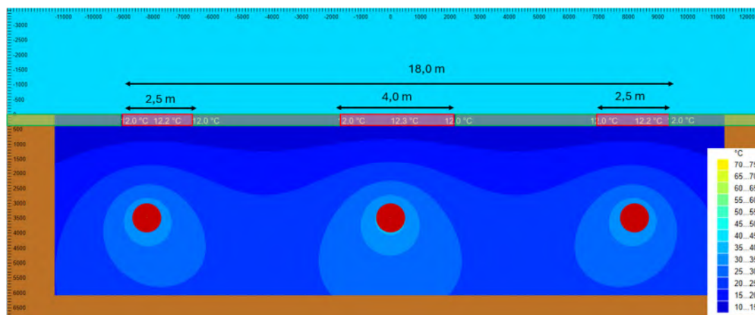
Figuur 18. Bodemtemperatuurprofiel voor een DN1200 waterstofleiding.
