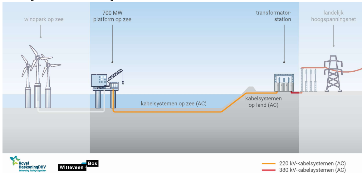
Afbeelding 1.3 – Schematische weergave van het elektriciteitsnet (wisselstroom).
