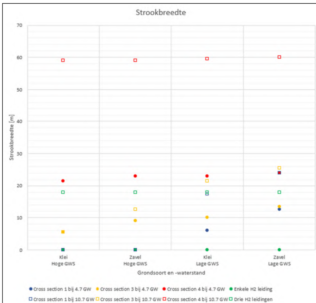
Figuur 20. Maximale strookbreedtes t.o.v. grondslagen en - waterstanden voor de verschillende configuraties..
