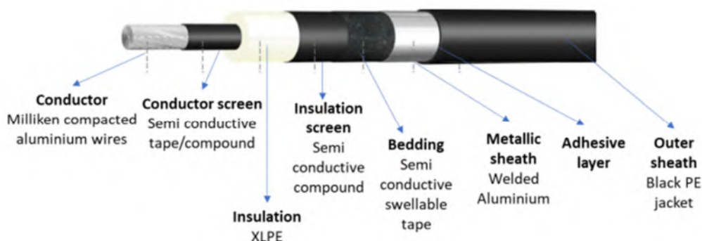
Figuur 2. Kabelopbouw AC kabel EYAKrvlwd.
