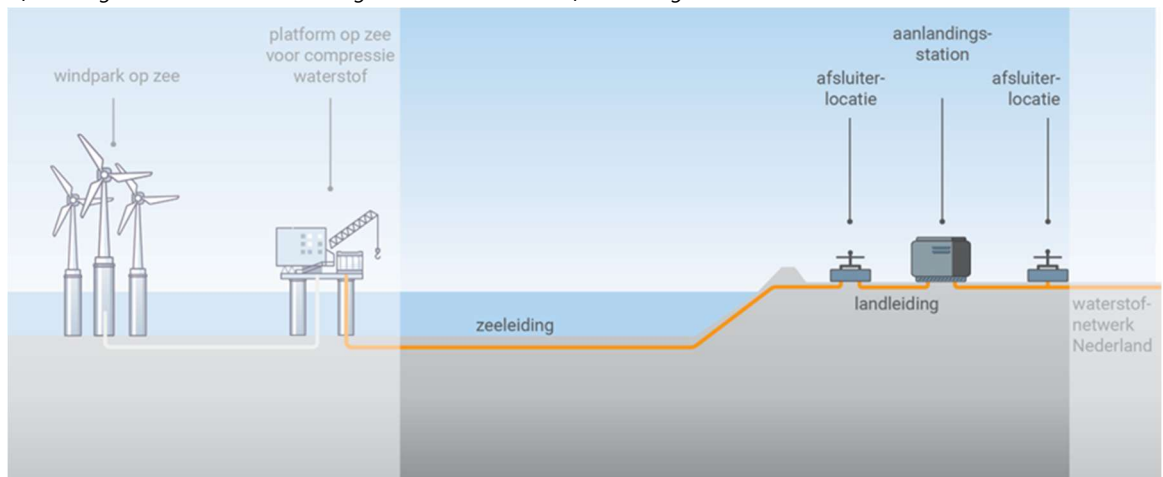
Afbeelding 1.4 - Schematische weergave van een waterstofverbinding
