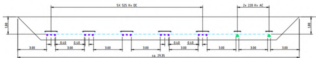
Figuur 6 - Kabelcorridor cross section 1 voor 10,7 GW scenario.
