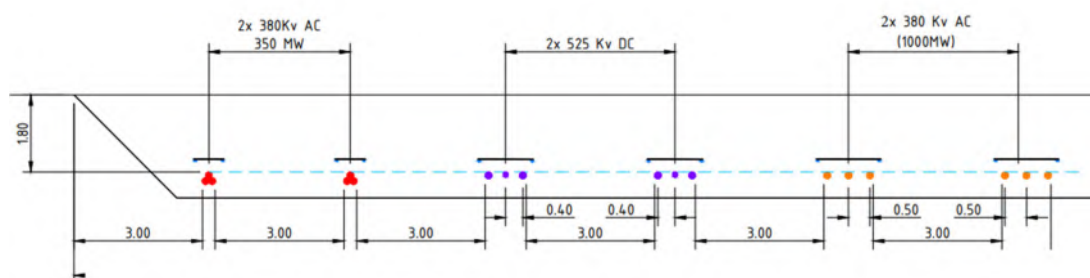
Figuur 9 – Kabelcorridor cross section 4 voor 4,7 GW scenario.
