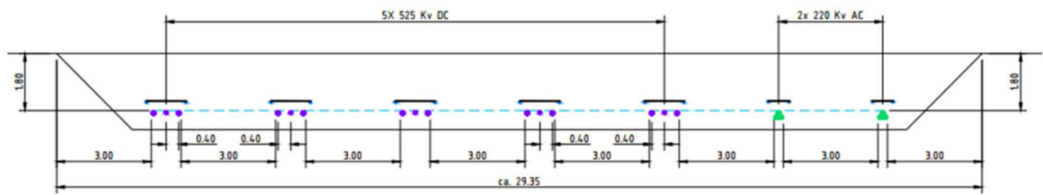
Afbeelding 6.7 - 'Cross section 1 10,7GW': toegepast als maatgevende configuratie voor de maximale scope van 7 kabels.
