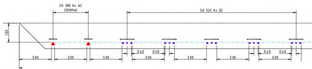
Figuur 8 - Kabelcorridor cross section 3 voor 10,7 GW scenario.
