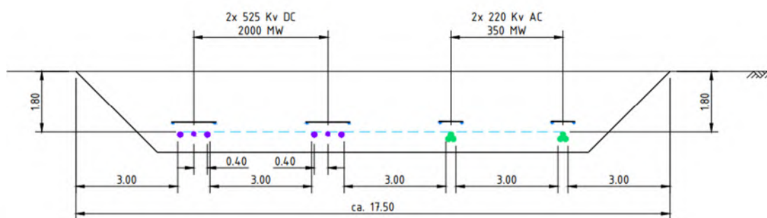
Figuur 5 – Kabelcorridor cross section 1 voor 4,7 GW scenario.
