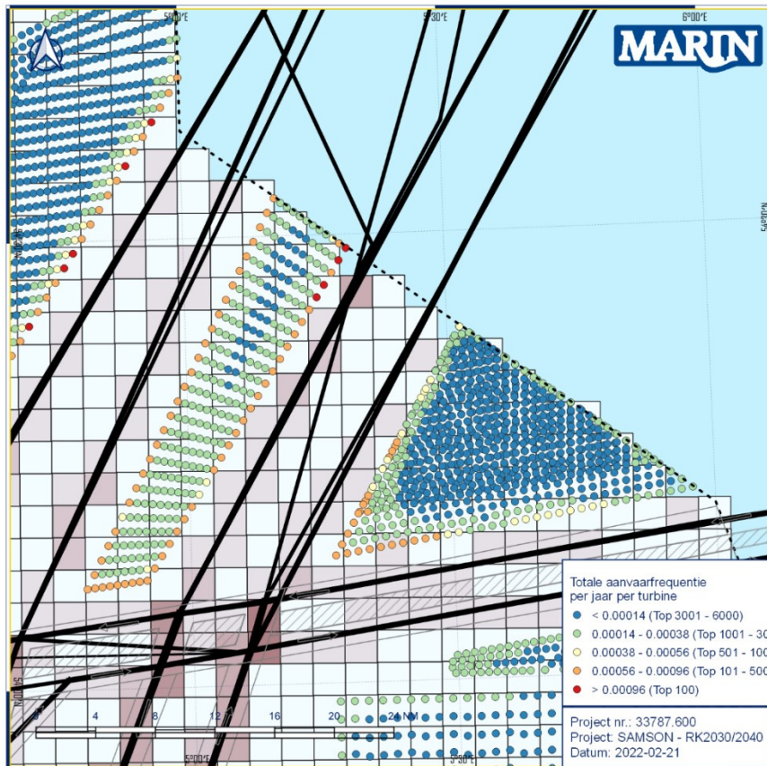
Figuur 4-18 Visualisatie aanvaringfrequentie per windturbine in windpark Doordewind [Ref 4.]
