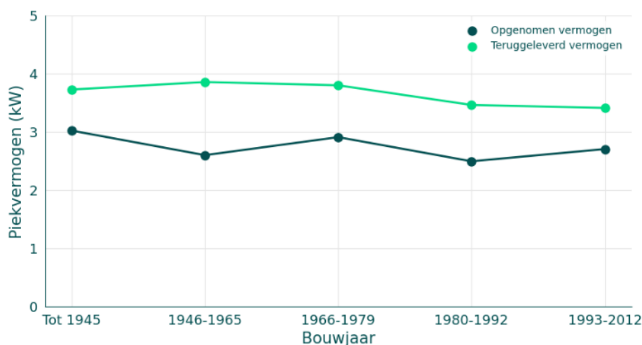
Figuur 4.2: Gelijktijdig piekvermogen van 1298 woningen met all-electric warmtepompen geclusterd op bouwperiode
