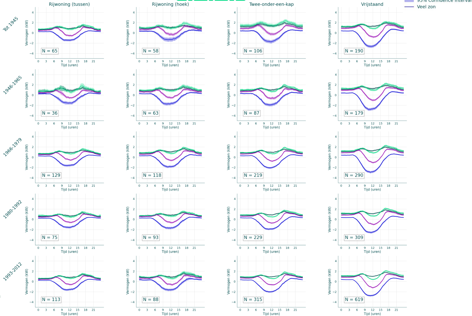
Figuur B.5 Dagprofielen referentieweken woningen met hybride warmtepomp (clusters: bouwperiode, woningtype)
