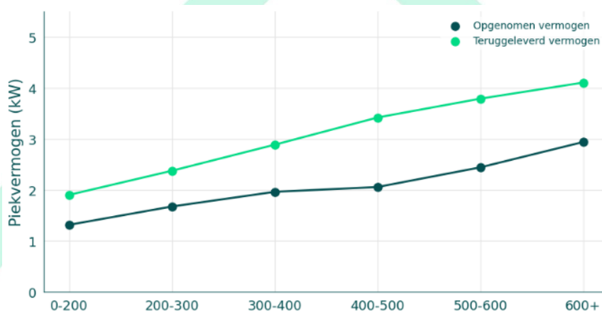
Figuur 4.5: Gelijktijdig piekvermogen van 3648 woningen met hybride warmtepompen geclusterd op verliesoppervlak
