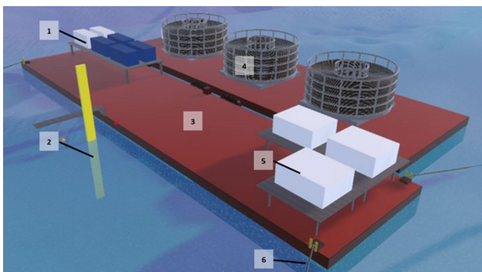
Figuur 3-14 - Schematisch overzicht van installatie door middel van een Vertical Injector
