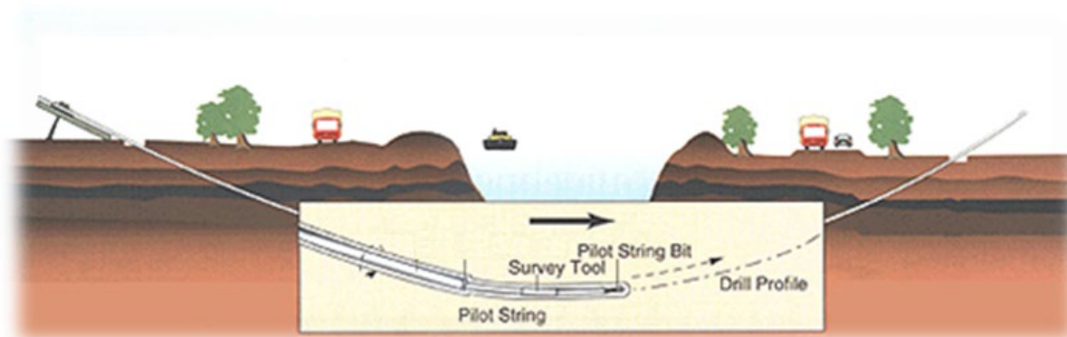
Figuur 52 Pilotfase
