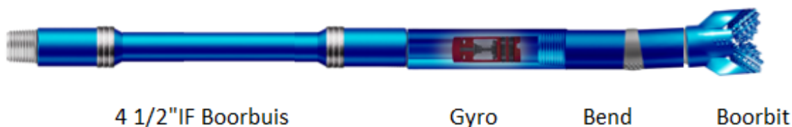
Figuur 53 Boorbit configuratie
