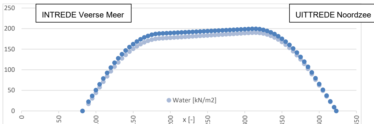
Figuur 6 Statische waterdruk en boorvloeiستفدرك in de boorgang HDD's IJmuiden Ver Alpha en Nederwiek 1
