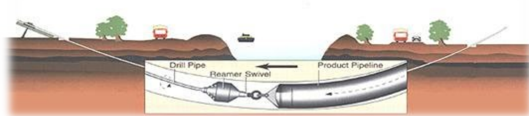
Figuur 55 Intrekfase
