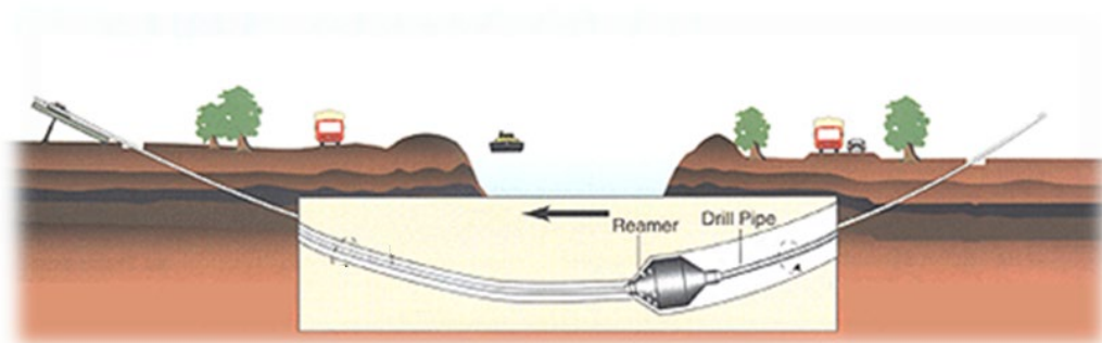
Figuur 54 Ruimfase
