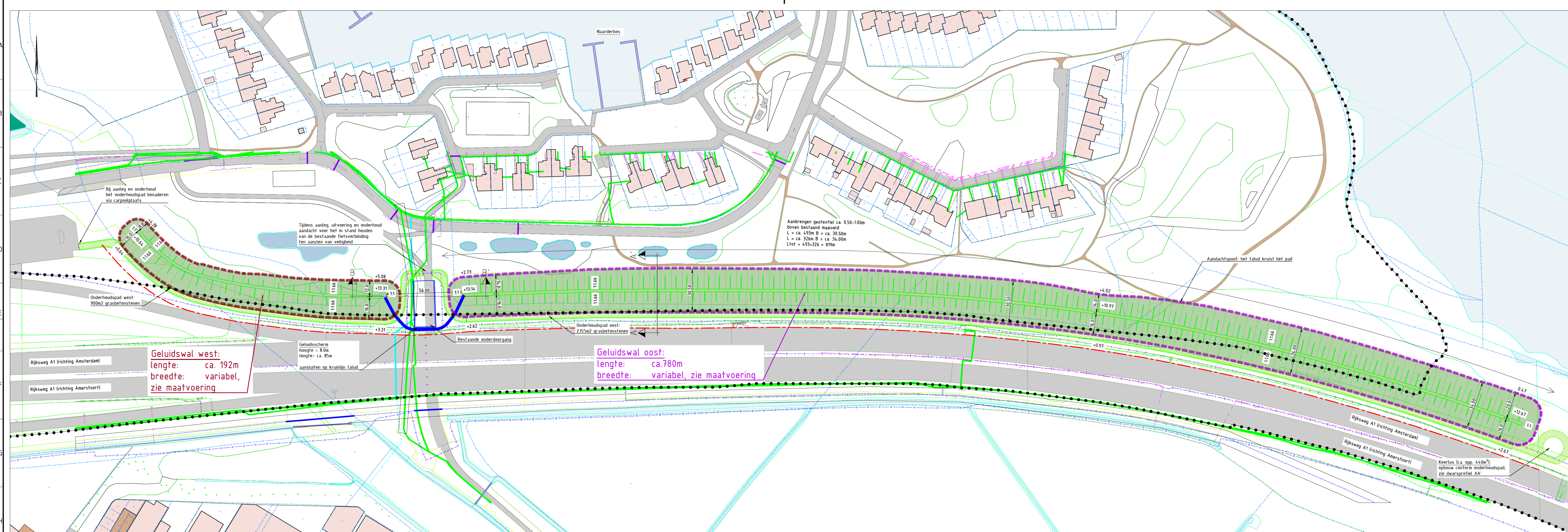
Situatieoverzicht: 1:1000
