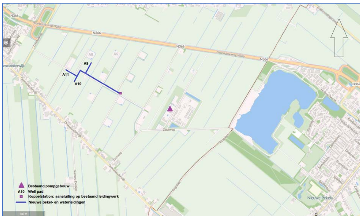
Figuur 2.3 Tracé transportleidingen water en pek (bron: MER HyStock)
