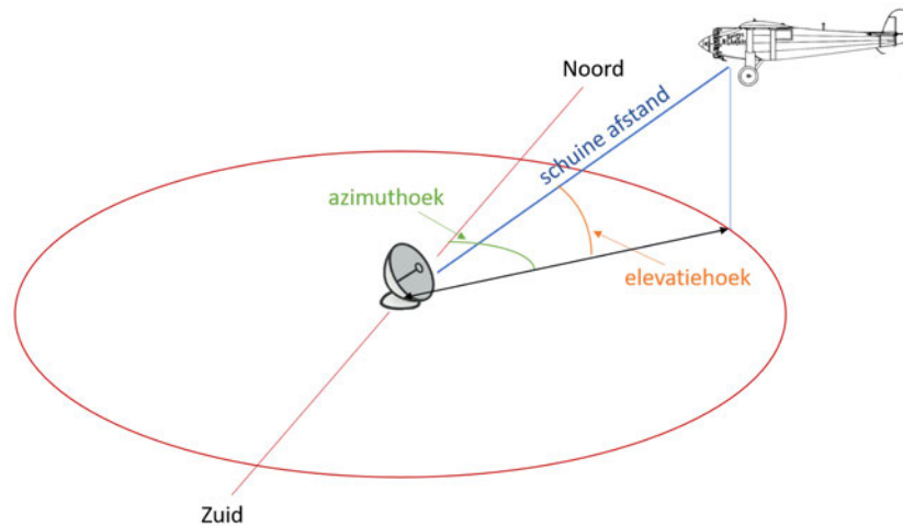
Figuur 2: Illustratie van de begrippen schuine afstand, azimuthhoek en elevatiehoek. De elevatiehoek is de hoek in het verticale vlak. De azimuthhoek is de hoek in het horizontale vlak ten opzichte van het noorden.
