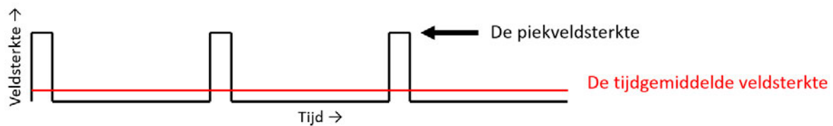
Figuur 5 : Schematische weergave van het uitgezonden signaal van de radar. Na de uitzending van de puls volgt een tijd waarin de radar luistert naar eventueel terugkomende pulsen. ICNIRP schrijft voor dat zowel de piekveldsterkte als de tijdgemiddelde veldsterkte moet worden getoetst.
