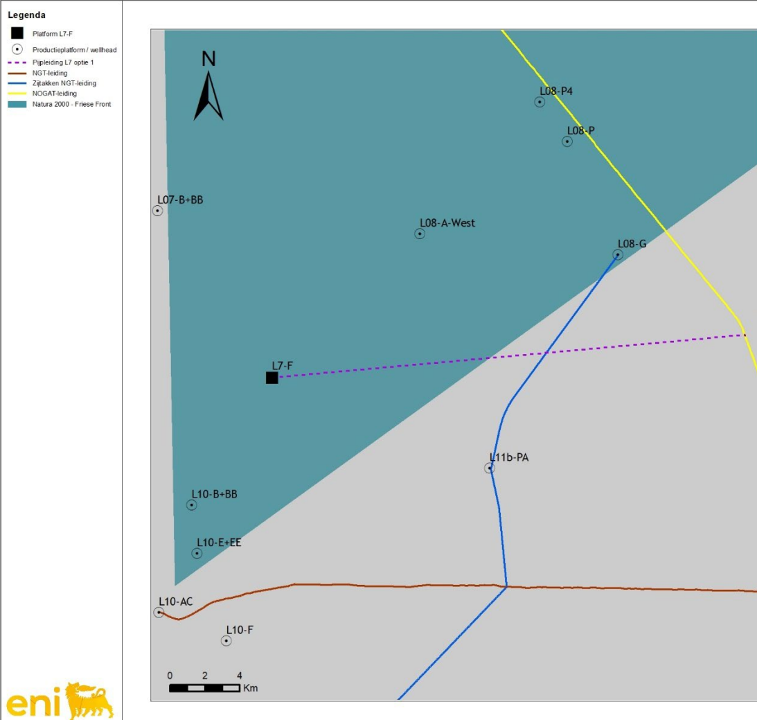
Figuur 1 Overzichtskartaat project gaswinning L7-F
