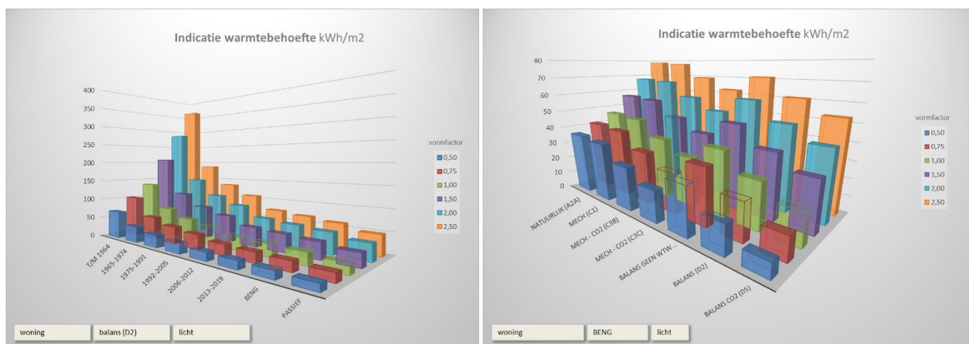
Figuur 2 Berekende warmtebehoefte woningen afhankelijk van vormfactor, ventilatiesysteem, bouwmasa (licht, zwaar) en isolatiegraad
