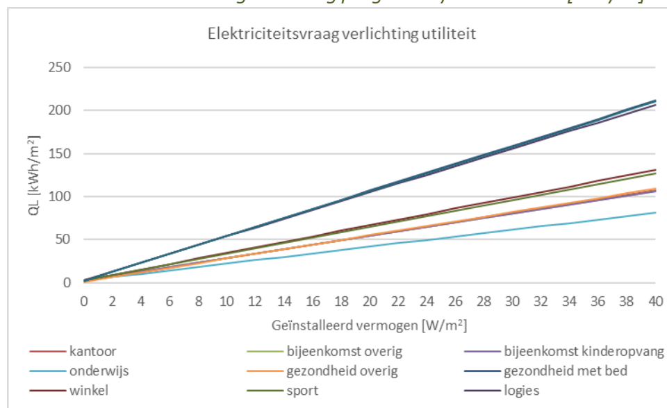
Figuur 5 Berekende elektriciteitsvraag verlichting per gebruiksfunctie utiliteit [kWh/m 2 ]
