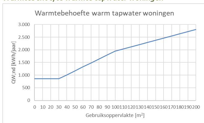
Figuur 4 Warmtebehoefte warmte tapwater woningen
