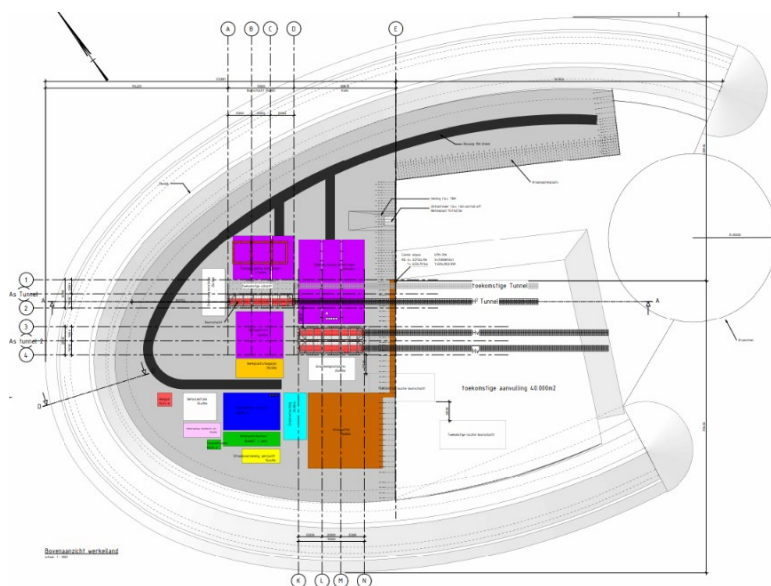
Afbeelding 6.3 Boven-aanzicht van intredepunt Noordzee van de X: Tunnelroute tijdens de bouwfase
