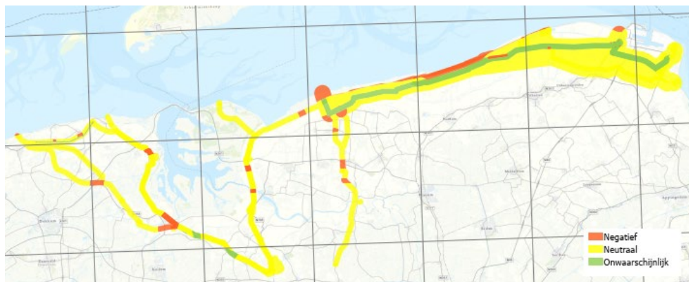
Afbeelding 7.5 NGE en munitiestort op de routes op land (REASeuro, 2024)
