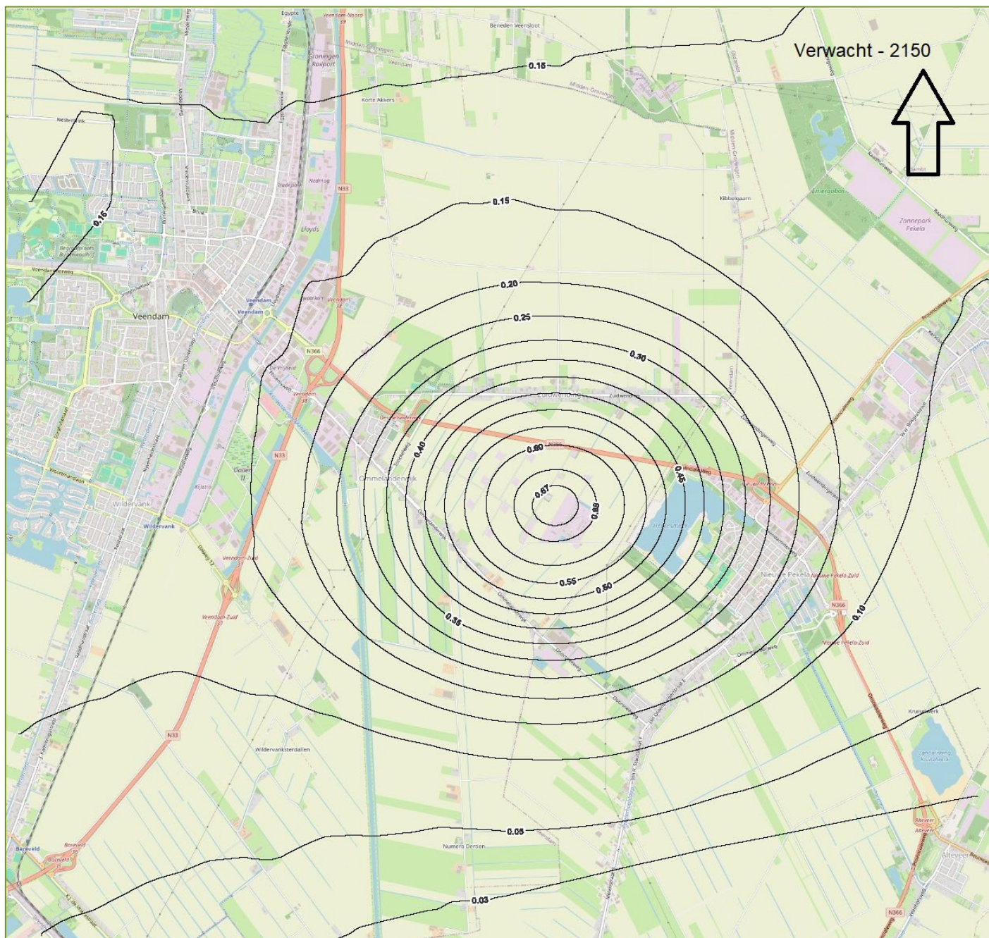
Figuur 7-9: Verwachte bodemdaling voor 2150 in m. (H2-max)
