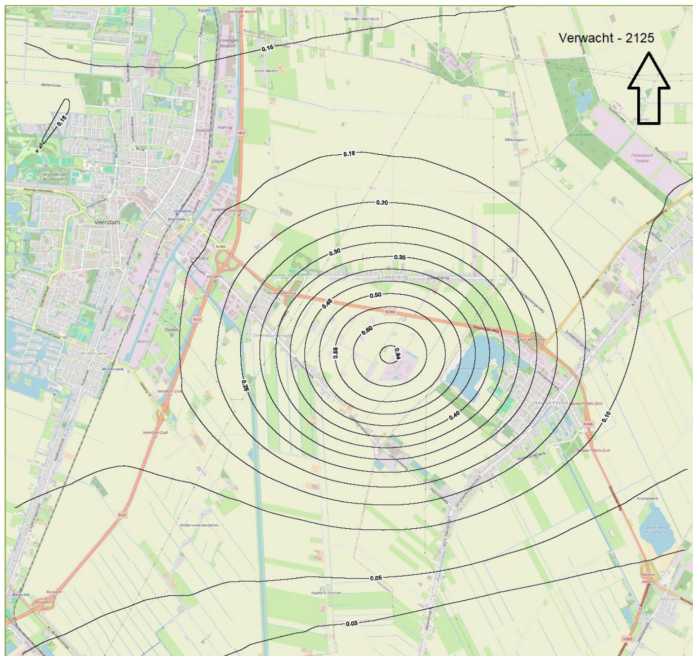
Figuur 7-8: Verwachte bodemdaling voor 2125 in m. (H2-max)
