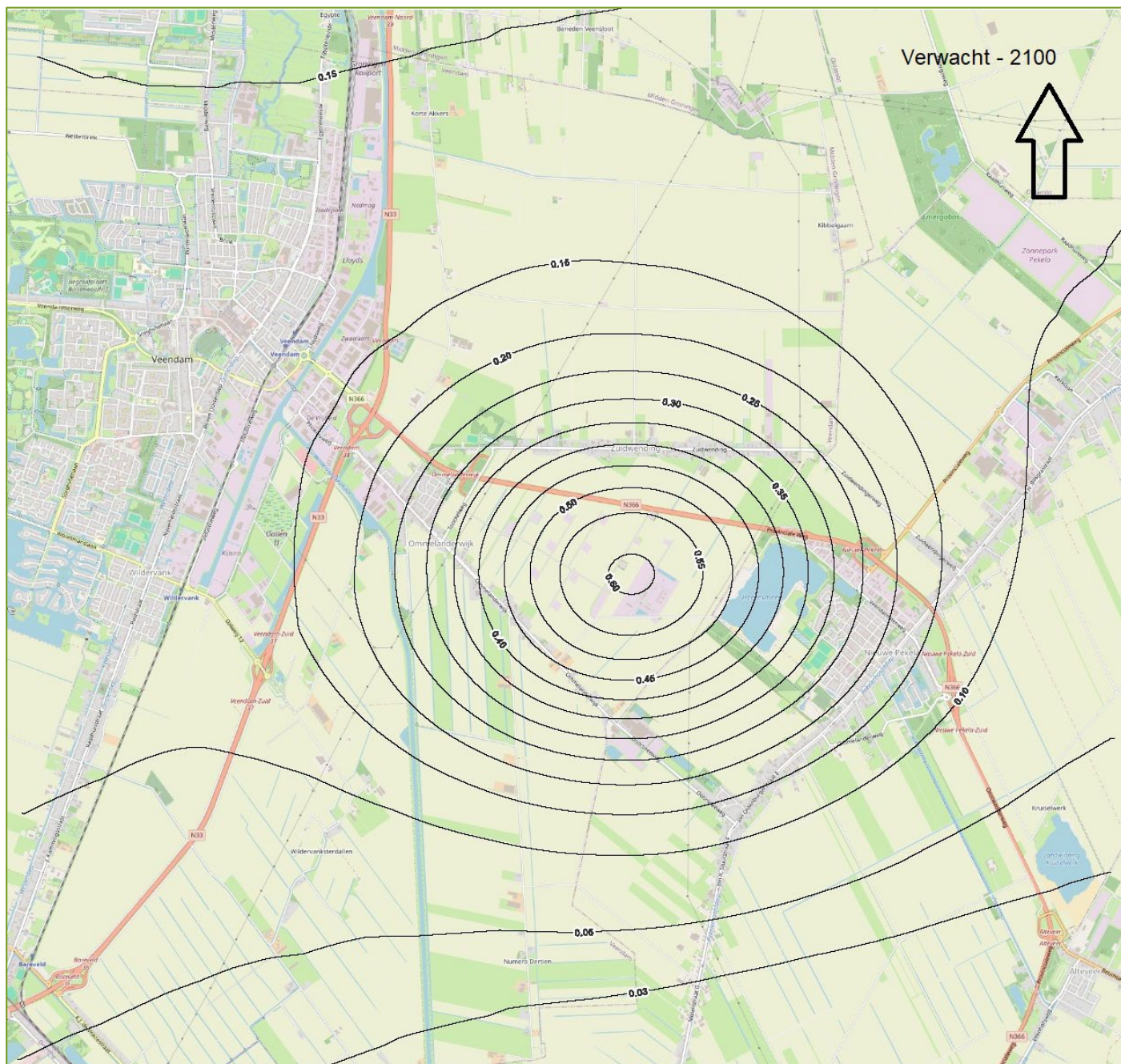
Figuur 7-7: Verwachte bodemdaling voor 2100 in m. (H2-max)
