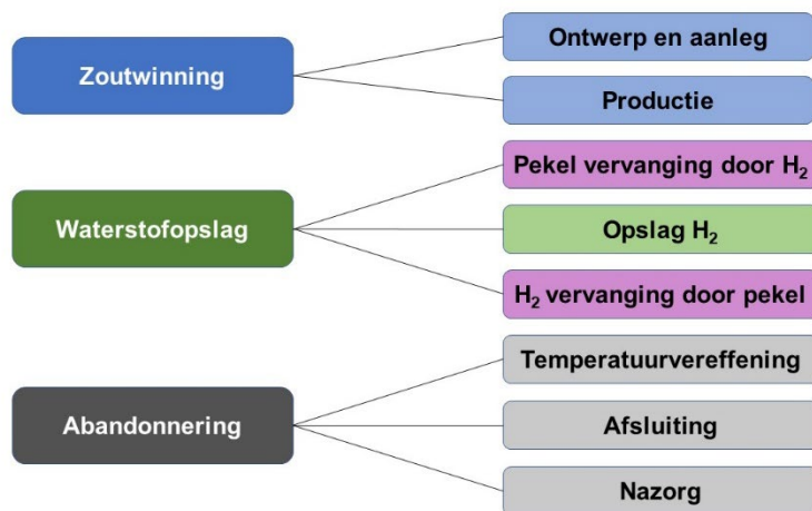
Figuur 2-2: Projectfasen.
