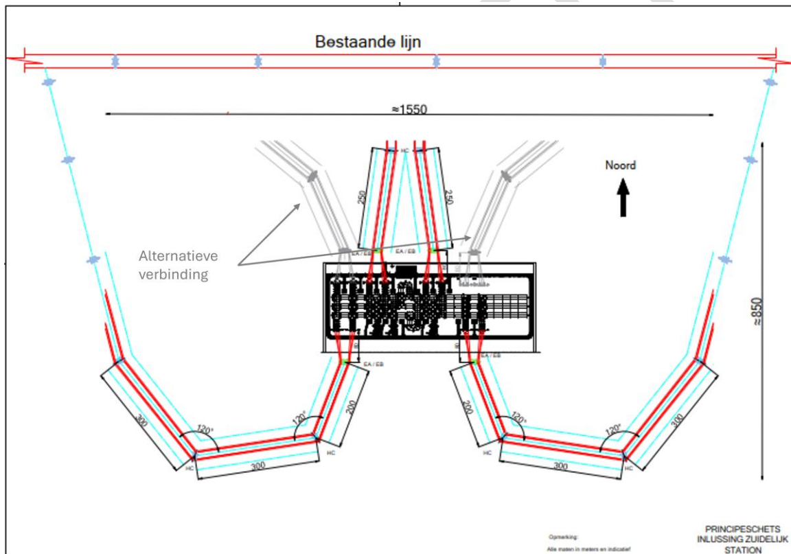
Afbeelding 4.3 Opstelling 2, indicatieve weergave parallel zuidelijk 380 kV-station
