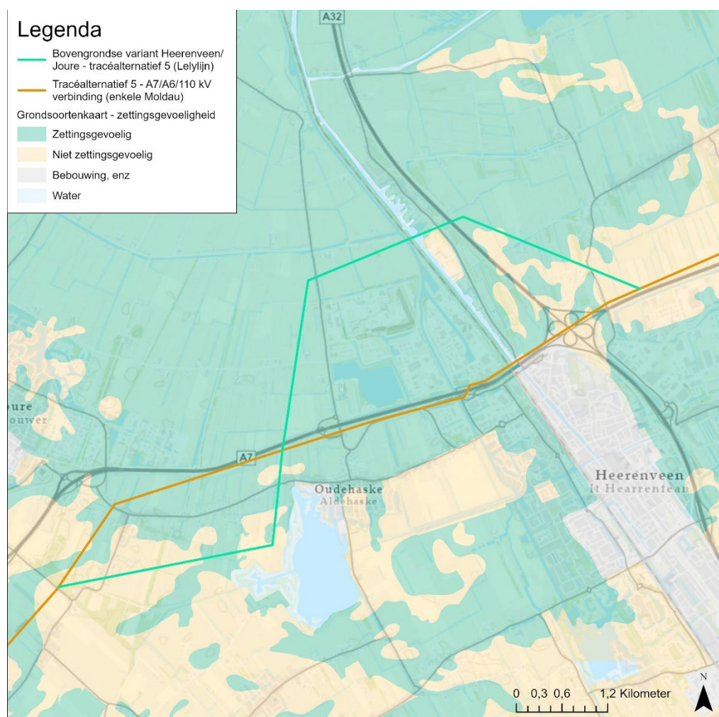
Figuur 5.17 Zettingsgevoeligheid bovengrondse variant Heerenveen/Joure (tracéalternatief 5)
