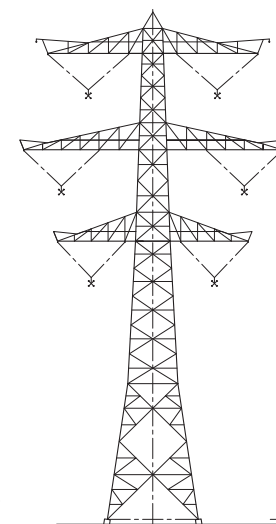
Figuur 2: Moldaumast
