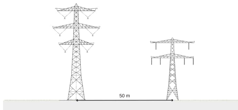
Afstand tussen een Moldaumast (links) en een bestaande verbinding (rechts)
