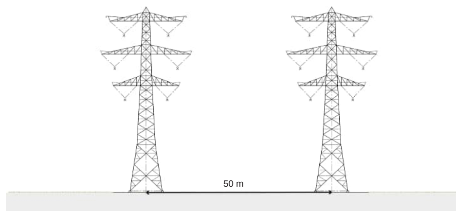
Afstand tussen twee parallel geplaatste Moldaumasten
