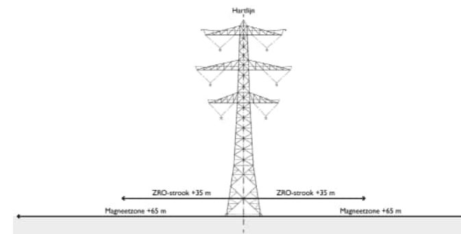
Positionering van een zakelijk rechtstrook rondom een enkele Moldaumas
