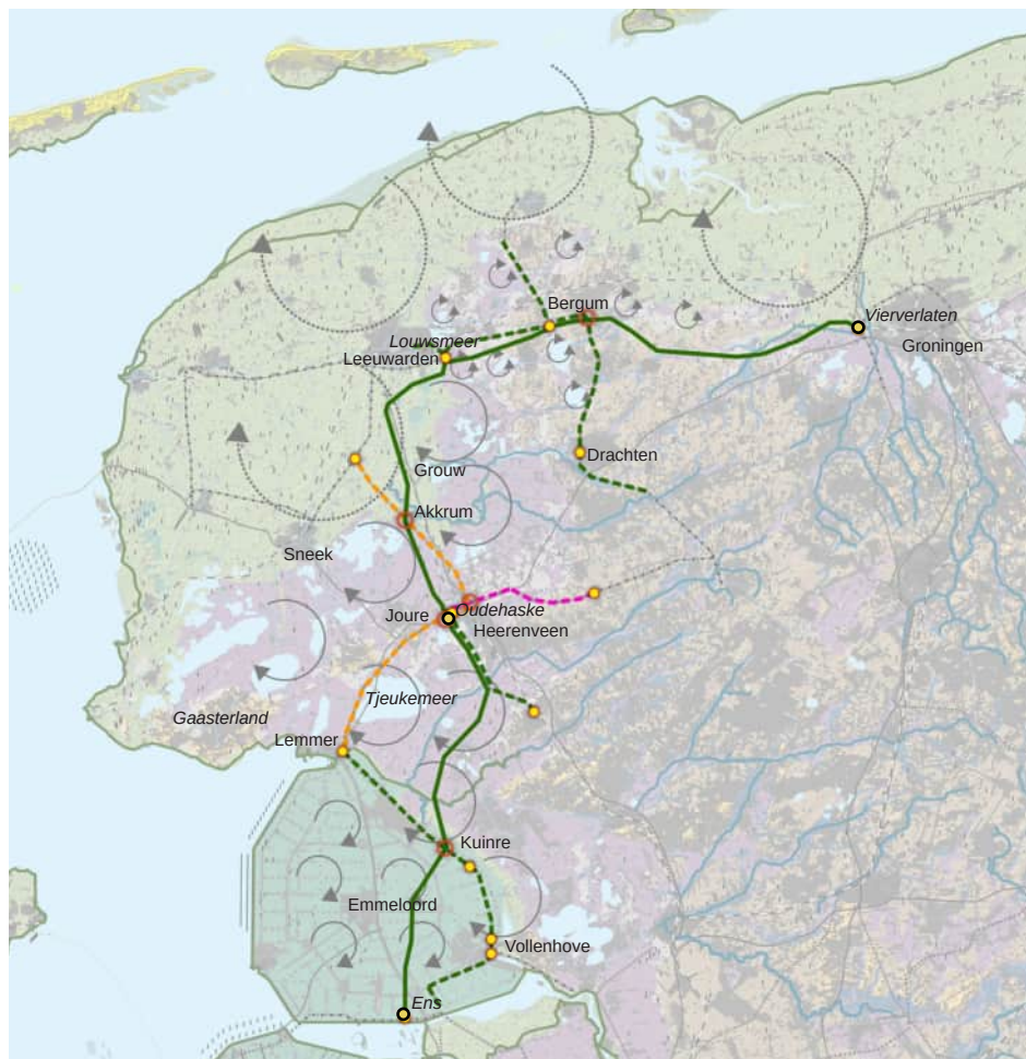
Figuur 23: Bestaande situatie hoogspanningsnetwerk in het studiegebied
