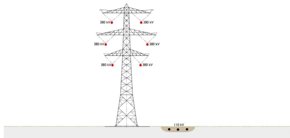
Combineren met bestaande 110 kV-hoogspanningsverbindingen, waarbij 110 kV wordt verkabeld
