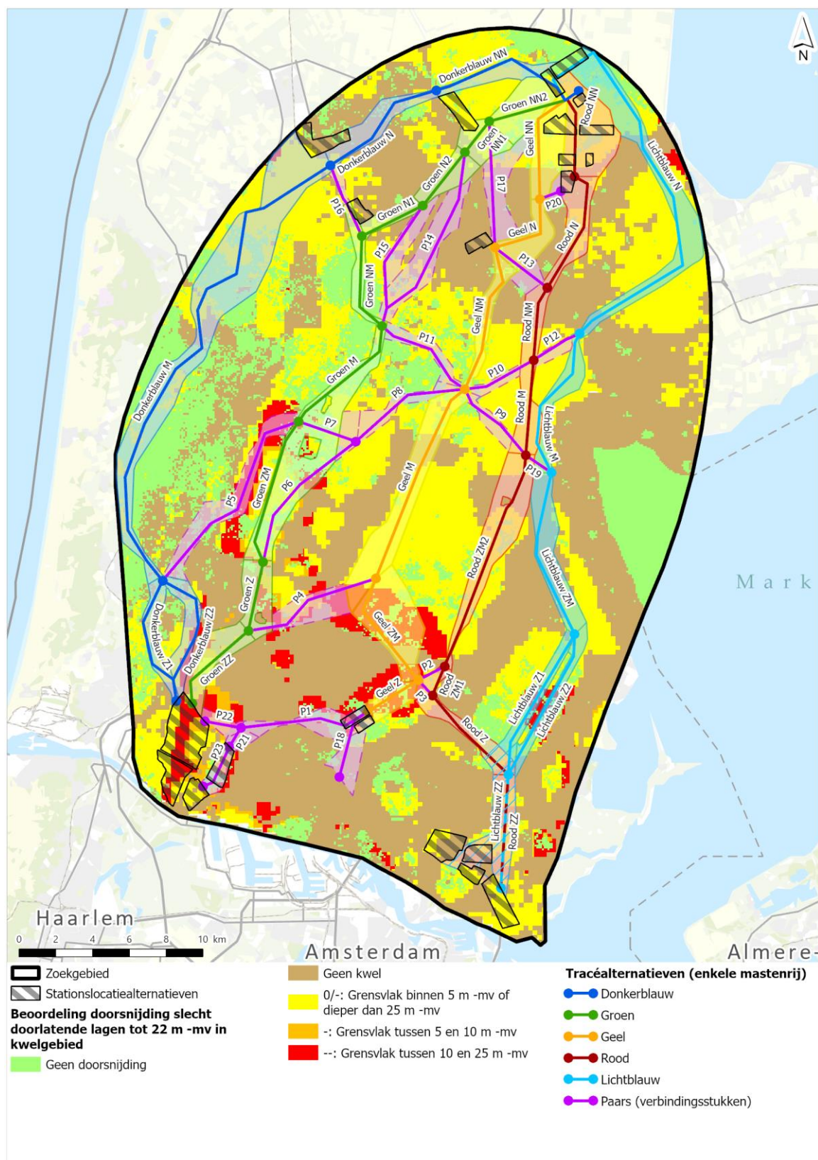
Afbeelding 5.4 Gebiedsdekkende beoordeling van effecten door veranderingen in grondwater door doorsnijding van slecht doorlatende lagen tot 22 m -mv in kwelgebieden - 380 kV-tracéalternatieven met één mastenrij
