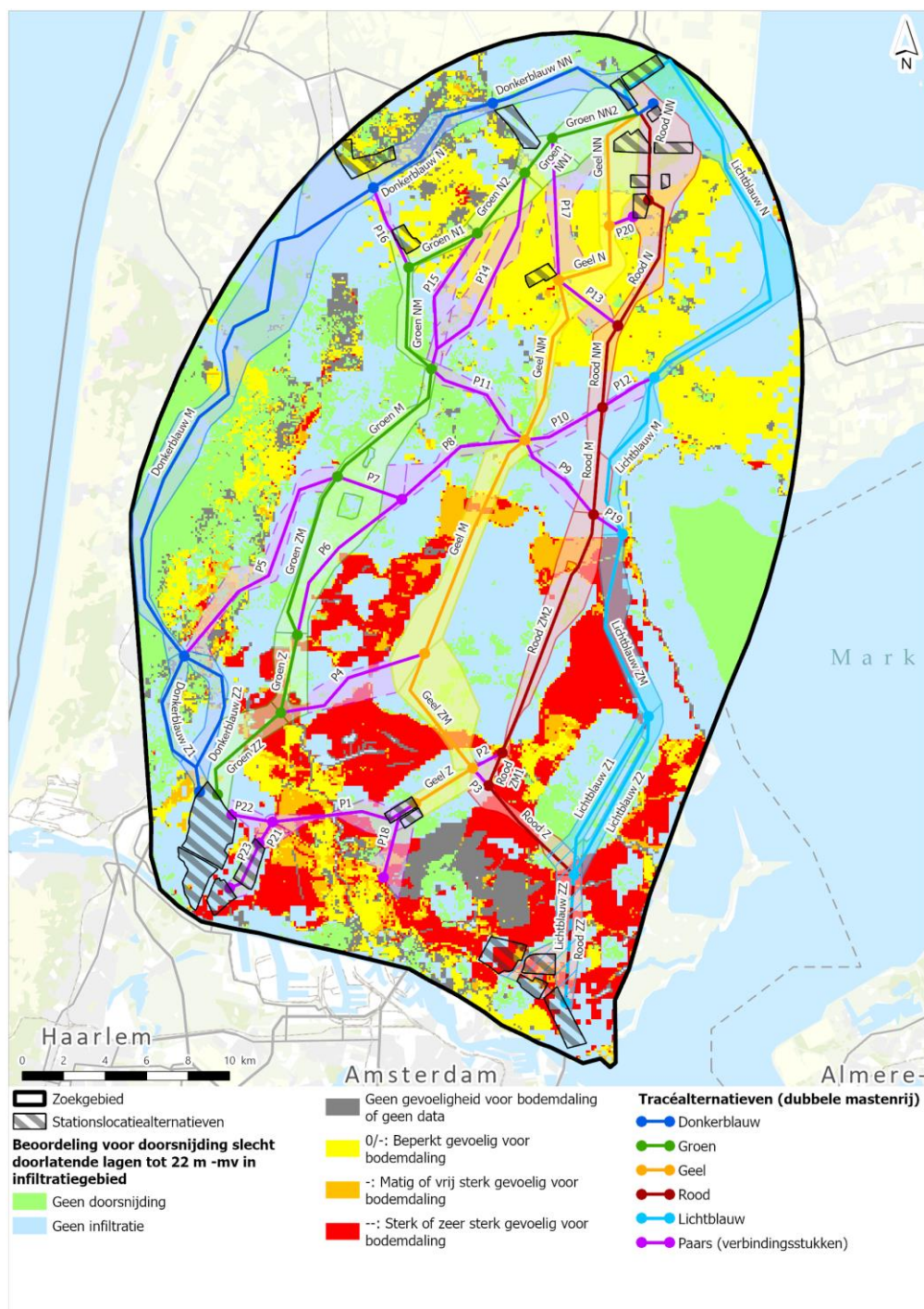
Afbeelding 6.5 Gebiedsdekkende beoordeling van effecten door veranderingen in grondwater door doorsnijding van slecht doorlatende lagen tot 22 m -mv in infiltratiegebieden - 380 kV-tracéalternatieven met twee mastenrijen
