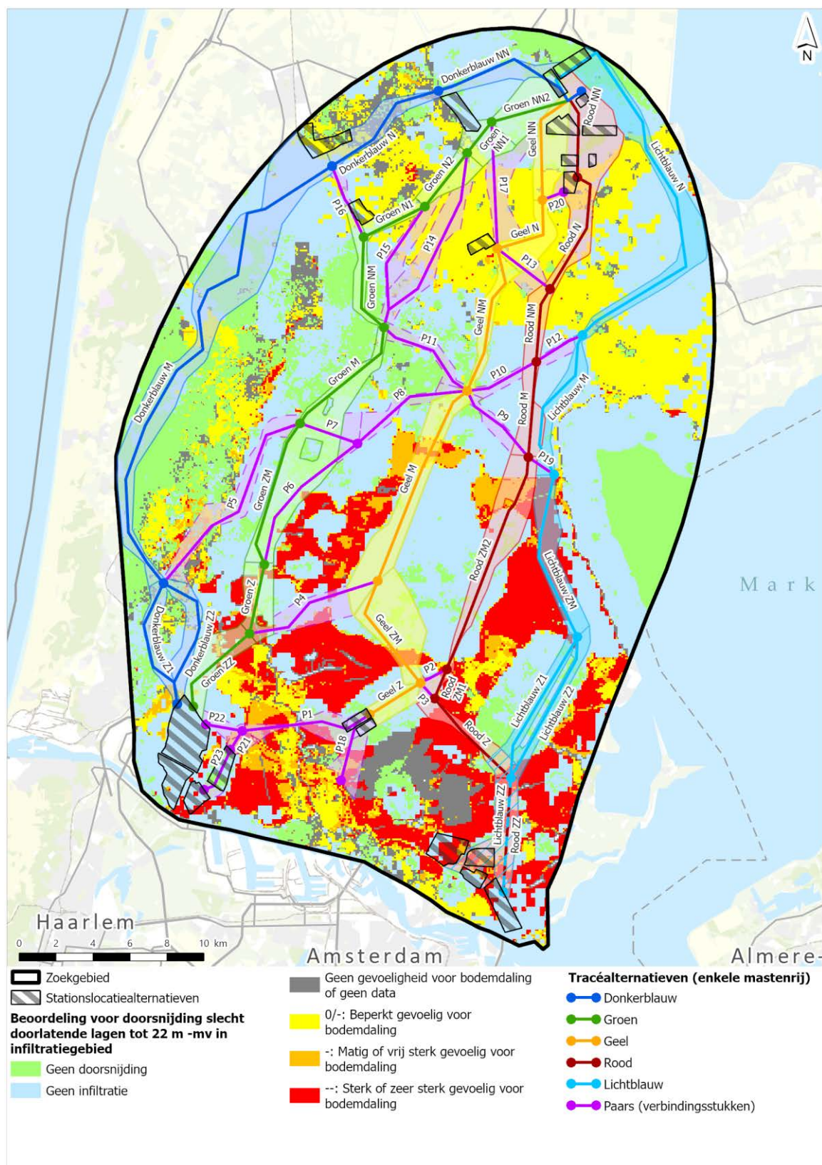
Afbeelding 5.5 Gebiedsdekkende beoordeling van effecten door veranderingen in grondwater door doorsnijding van slecht doorlatende lagen tot 22 m -mv in infiltratiegebieden - 380 kV-tracéalternatieven met één mastenrij
