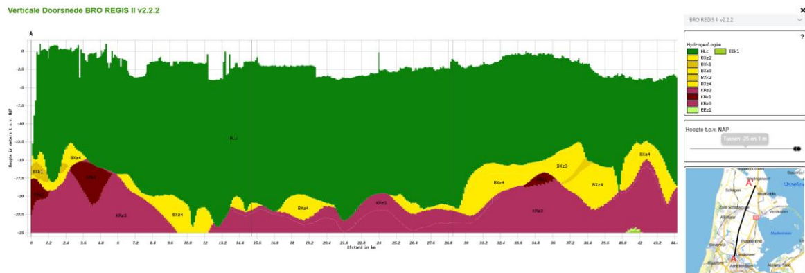
Afbeelding 3.2 Bodemopbouw over een zuid-noord doorsnede over het zoekgebied (bron: DINOloket - BRO REGIS II v2.2.2)
