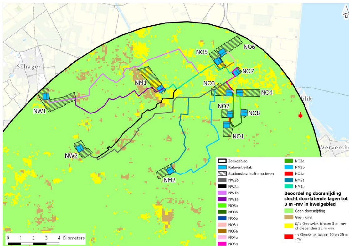
Afbeelding 8.4 Gebiedsdekkende beoordeling in het gebied van de ondergrondse tracéalternatieven, van effecten door veranderingen in grondwater door doorsnijding van slecht doorlatende lagen tot 3 m -mv in kwelgebieden - 150 kV-tracéalternatieven
