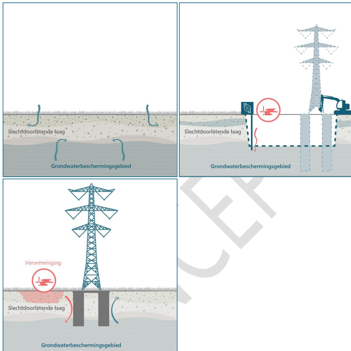
Afbeelding 5.7 De huidige situatie van het grondwaterbeschermingsgebieden (linksboven) en het effect van bemalingen (rechts) en gebruik (linksonder) van een 380 kV-hoogspanningsverbinding dat mogelijke verontreiniging van de drinkwaterbron kan veroorzaken
