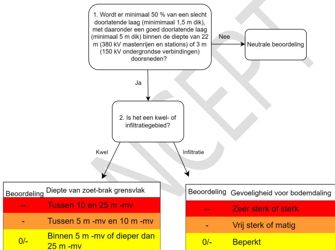
Afbeelding I.1 Diagram stappen beoordeling grondwaterkwantiteit
