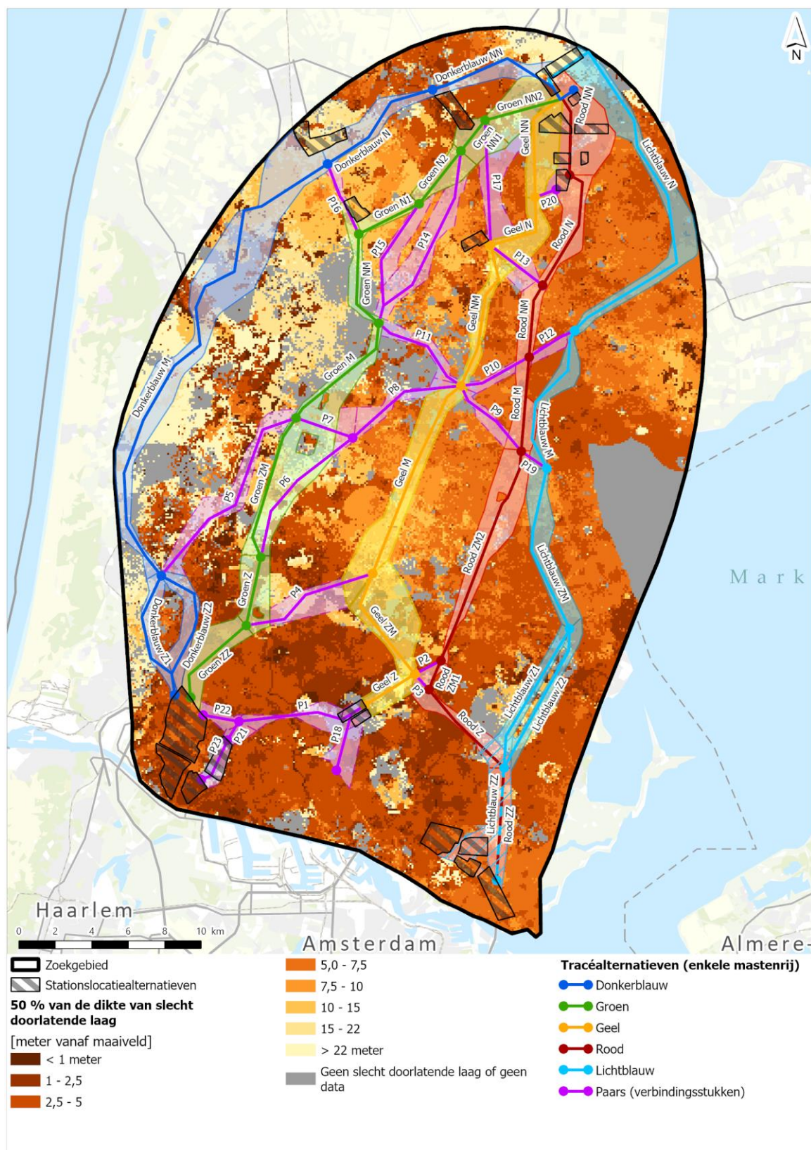
Afbeelding 5.3 50 % van de dikte van de bovenste slecht doorlatende laag vanaf het maaiveld ten opzichte van maaiveld - 380 kV-tracéalternatieven met één mastenrij
