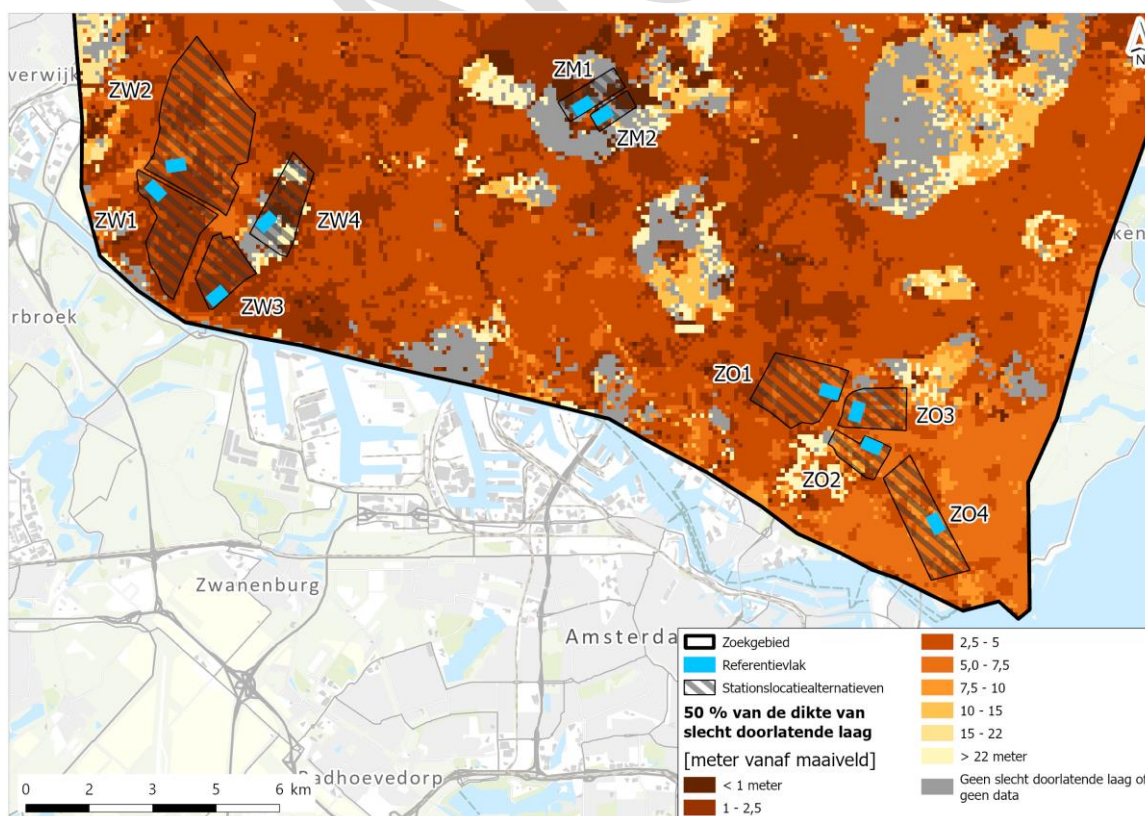
Afbeelding 7.4 50 % van de dikte van de eerste slecht doorlatende laag vanaf het maaiveld ten opzichte van maaiveld - zuidelijke stationslocatiealternatieven
