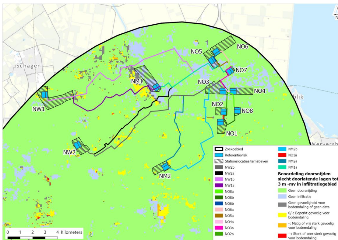
Afbeelding 8.5 Gebiedsdekkende beoordeling in het gebied van de ondergrondse tracéalternatieven, van effecten door veranderingen in grondwater door doorsnijding van slecht doorlatende lagen tot 3 m -mv in infiltratiegebieden - 150 kV-tracéalternatieven
