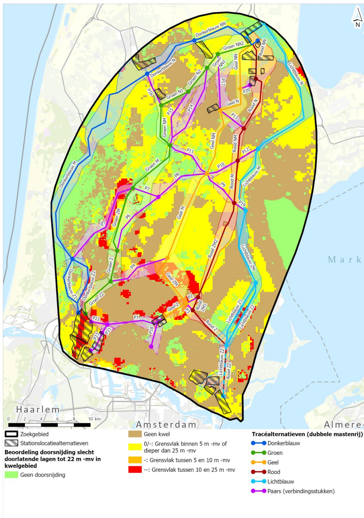
Afbeelding 6.4 Gebiedsdekkende beoordeling van effecten door veranderingen in grondwater door doorsnijding van slecht doorlatende lagen tot 22 m -mv in kwelgebieden - 380 kV-tracéalternatieven met twee mastenrijen
