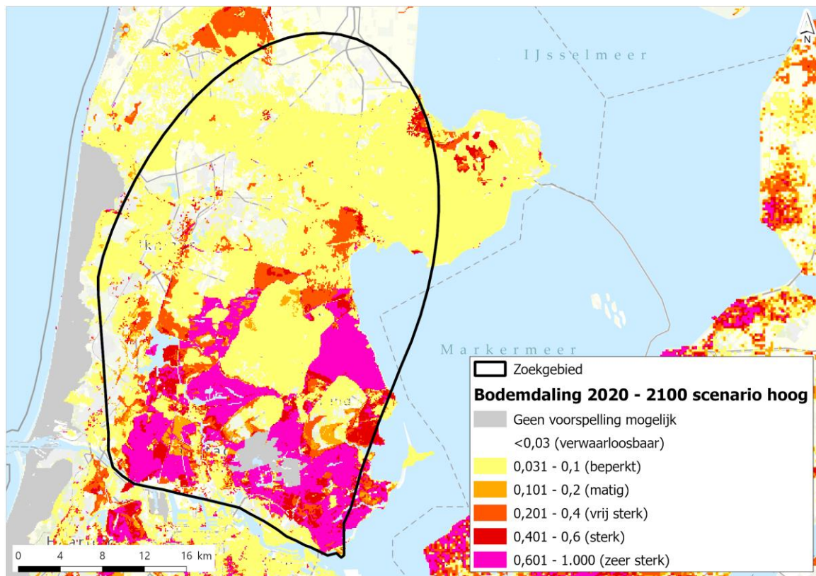
Afbeelding 3.6 Gevoeligheid voor bodemdaling in meters bij het scenario 2100 Hoog (bron: Klimaateffectatlas, 2025; Deltares, WEnR en TNO, 2021)
