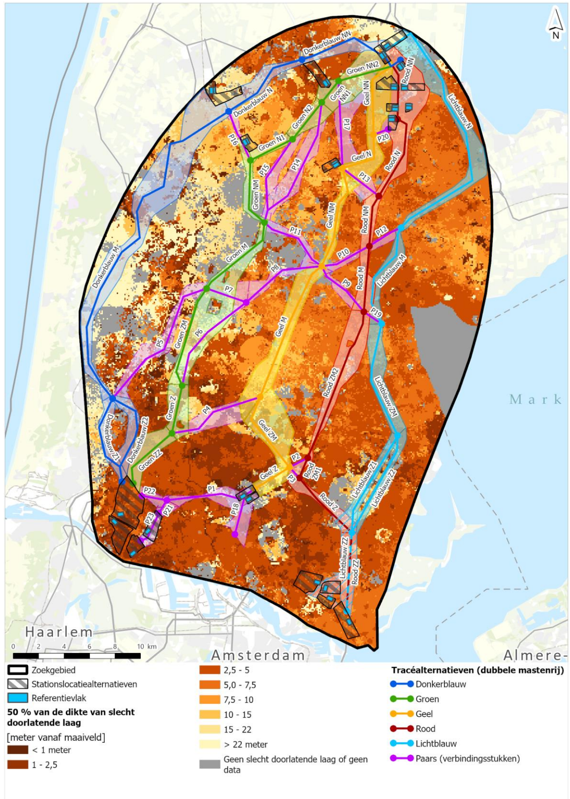
Afbeelding 6.3 50 % van de dikte van de bovenste slecht doorlatende laag vanaf het maaiveld ten opzichte van maaiveld - 380 kV-tracéalternatieven met twee mastenrijen
