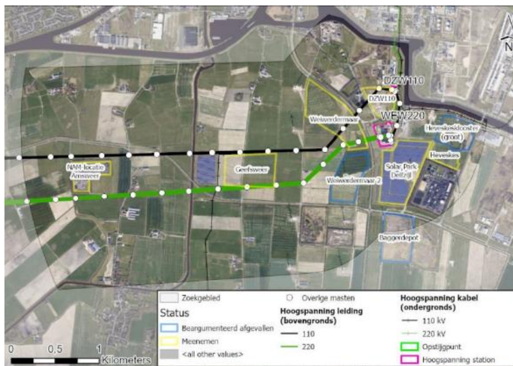
Figuur 0-1 Locatiealternatieven Hoogspanningsstation Farmsum (bron: Haalbaarheidsstudie)
