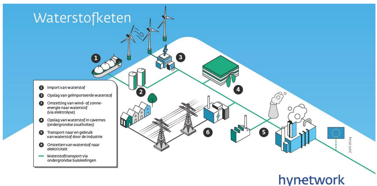
Figuur 6-3: Schematische weergave levering, transport en gebruik van waterstof (hogedruknetwerk) (bron: Hynetwork).
