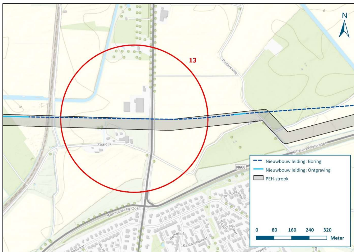
Figuur 15 | 13 Optimalisatie tracé Woensdrecht - Vlissingen
