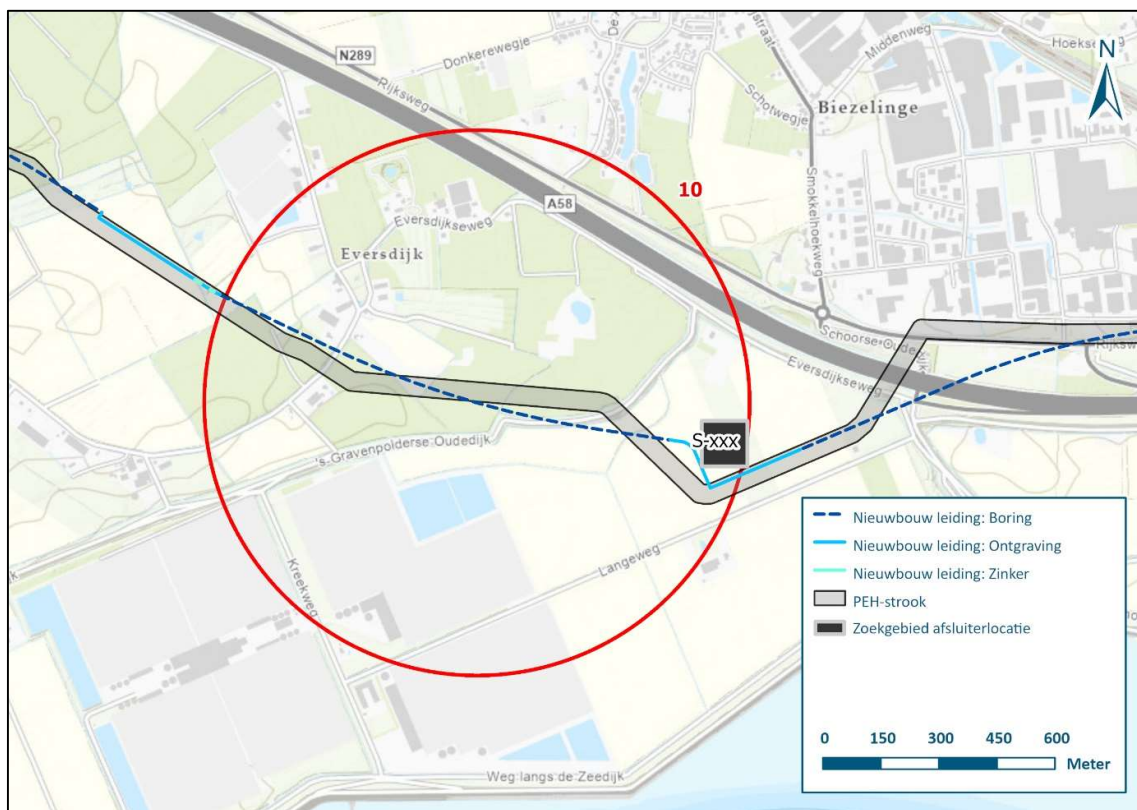
Figuur 12 | 10 Optimalisatie tracé Woensdrecht - Vlissingen
