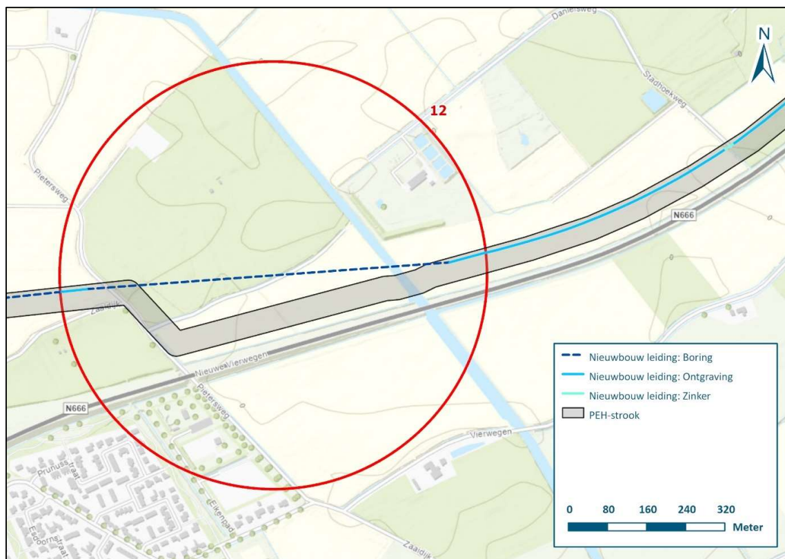
Figuur 14 | 12 Optimalisatie tracé Woensdrecht - Vlissingen
