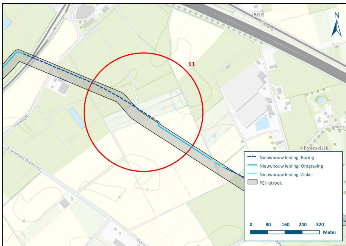
Figuur 13 | 11 Optimalisatie tracé Woensdrecht - Vlissingen
