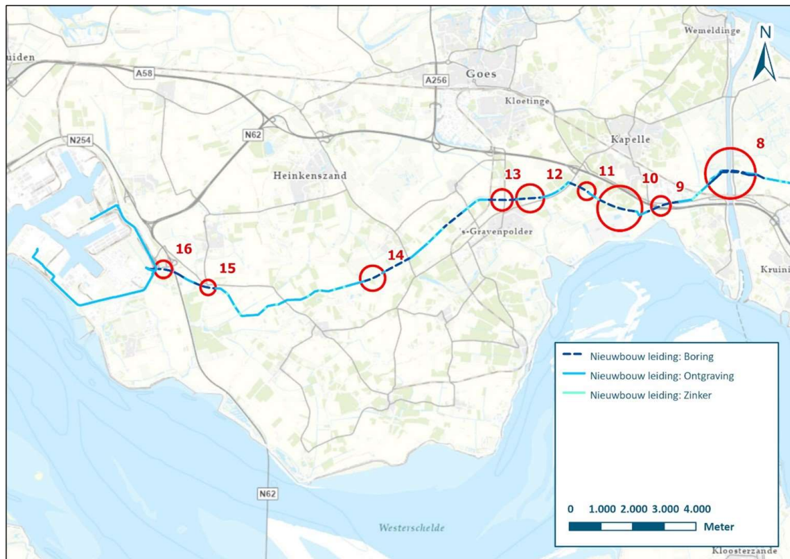
Figuur 2 | 02 - Overzichtskaart optimalisatie buisleidingstraat tracédeel Woensdrecht – Vlissingen (8tm16)
