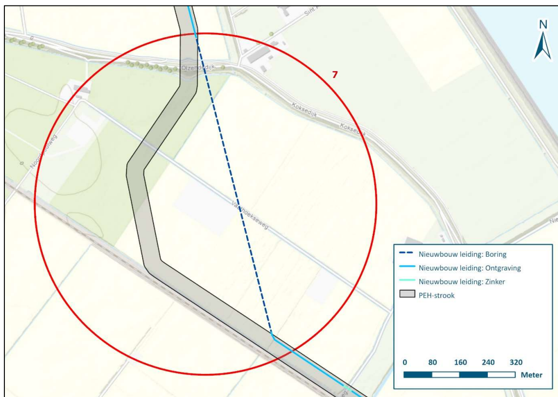
Figuur 9 | 07 Optimalisatie tracé Woensdrecht - Vlissingen
