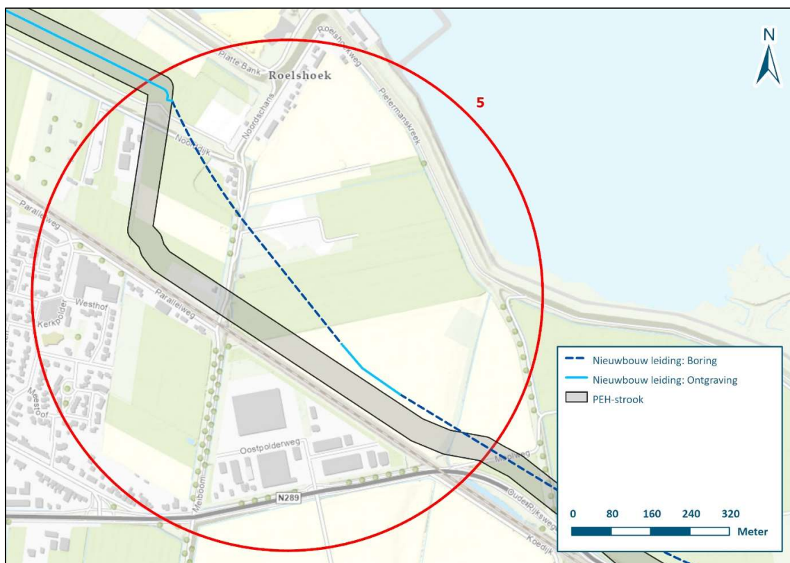
Figuur 7 | 05 Optimalisatie tracé Woensdrecht - Vlissingen
