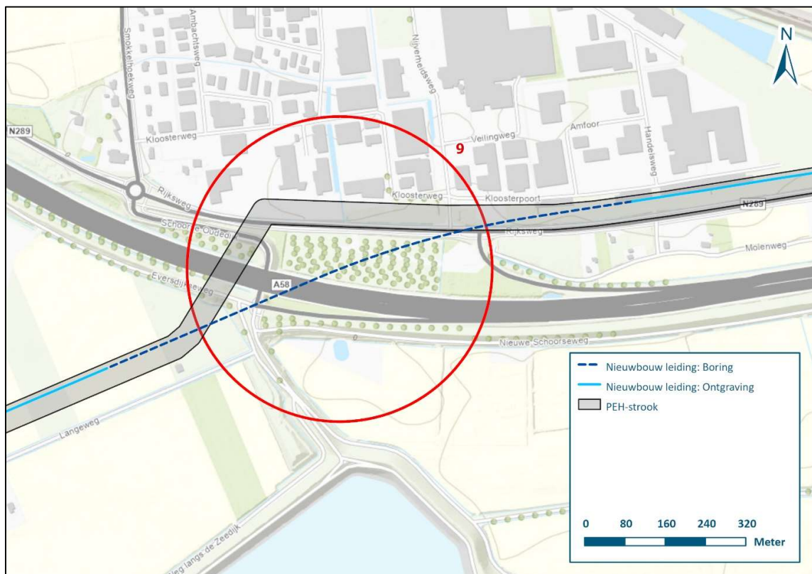
Figuur 11 | 09 Optimalisatie tracé Woensdrecht - Vlissingen
