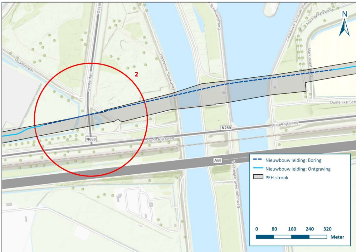
Figuur 4 | 02 Optimalisatie tracé Woensdrecht - Vlissingen
