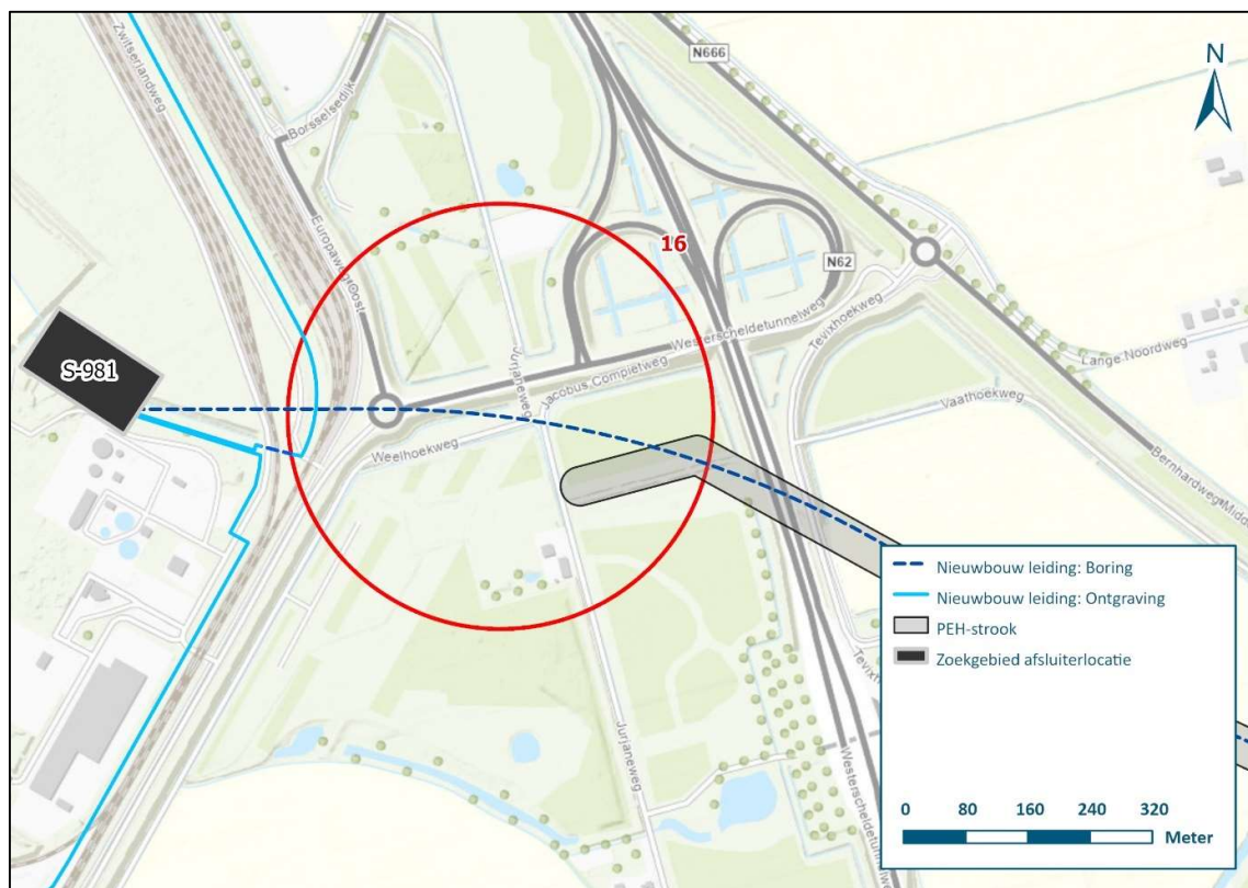
Figuur 18 | 16 Optimalisatie tracé Woensdrecht - Vlissingen
