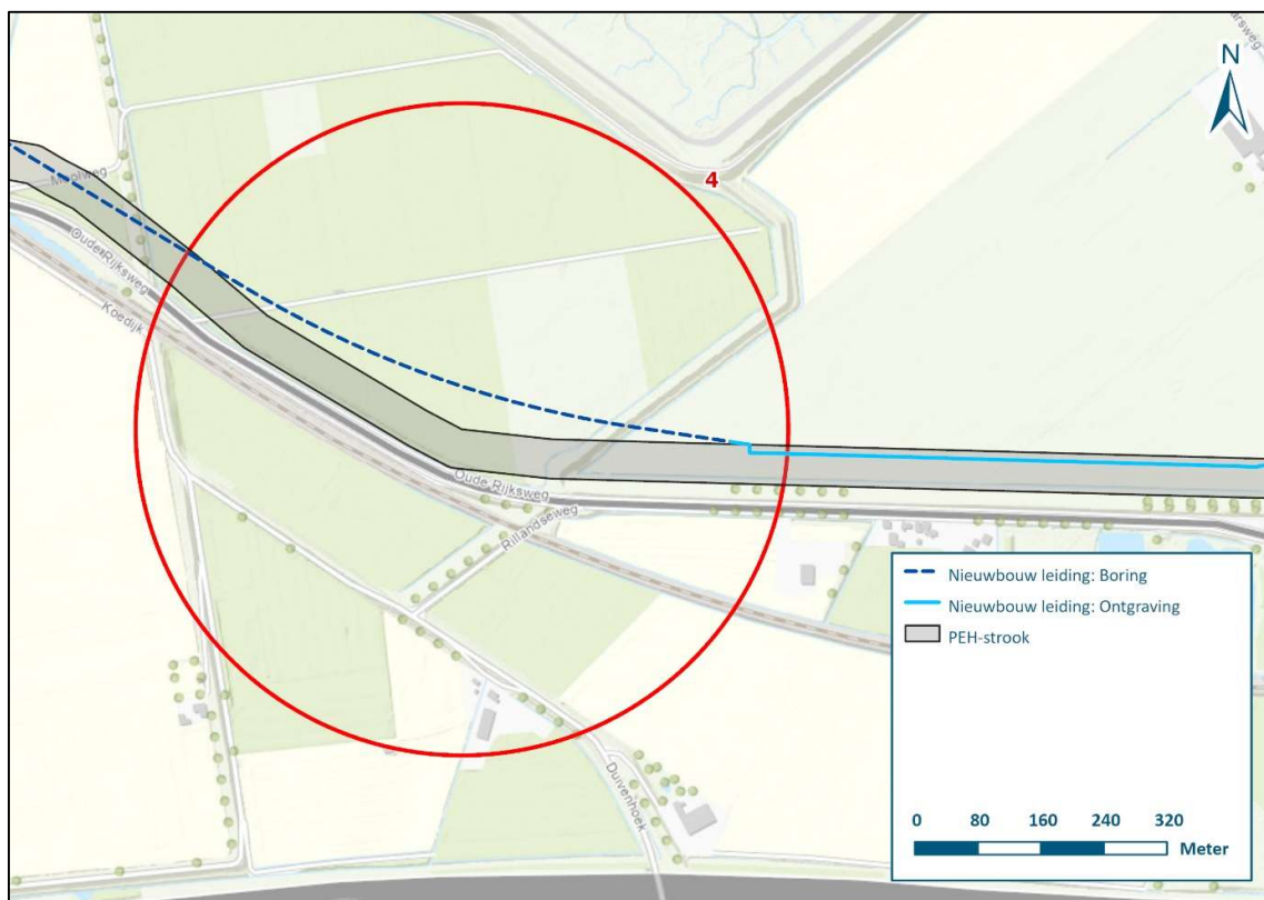
Figuur 6 | 04 Optimalisatie tracé Woensdrecht - Vlissingen
