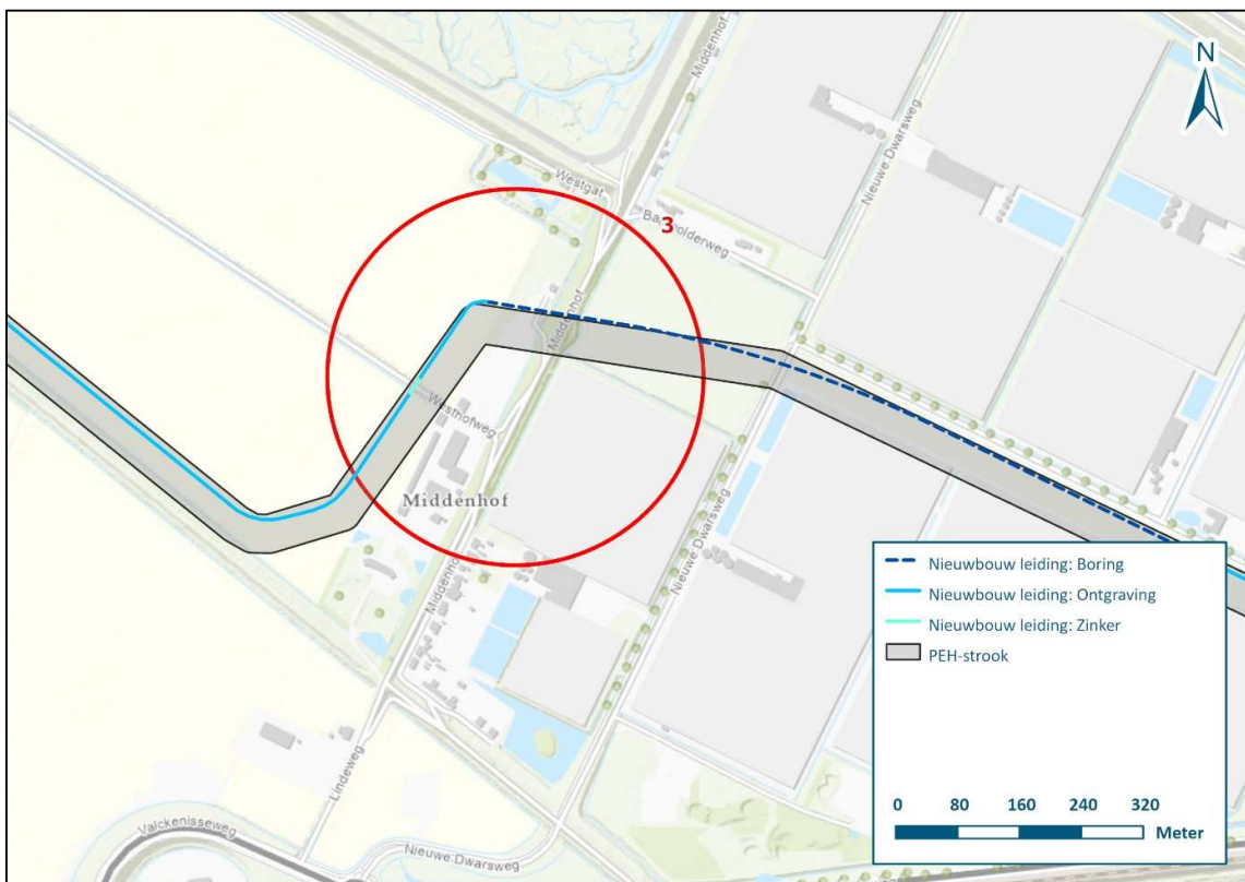
Figuur 5 | 03 Optimalisatie tracé Woensdrecht - Vlissingen
