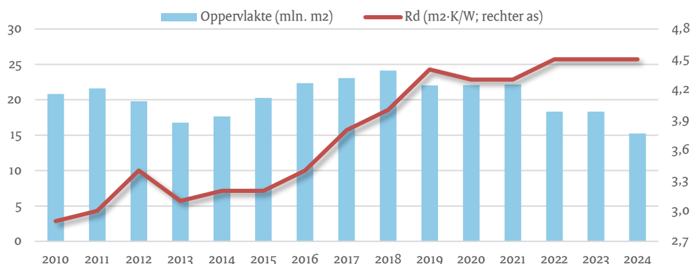
Grafiek 1: Totaal toepassing minerale en organische wullen in de bouwschil
