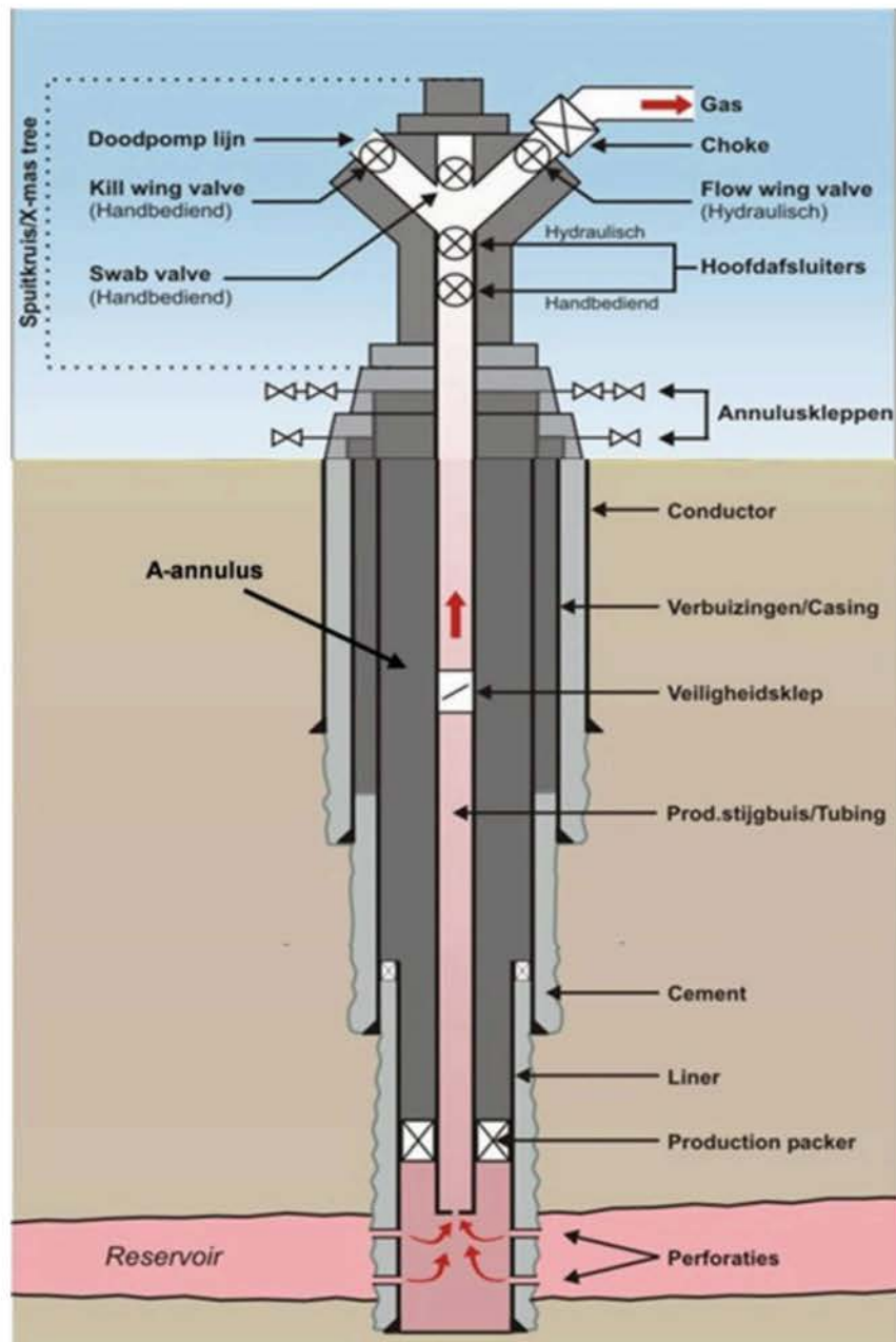
Schematische weergave van een put
