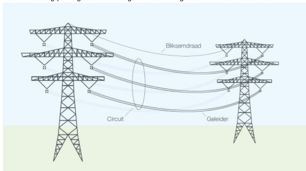
Figuur 44: Schematisch overzicht van de circuits in een hoogspanningsmast.
