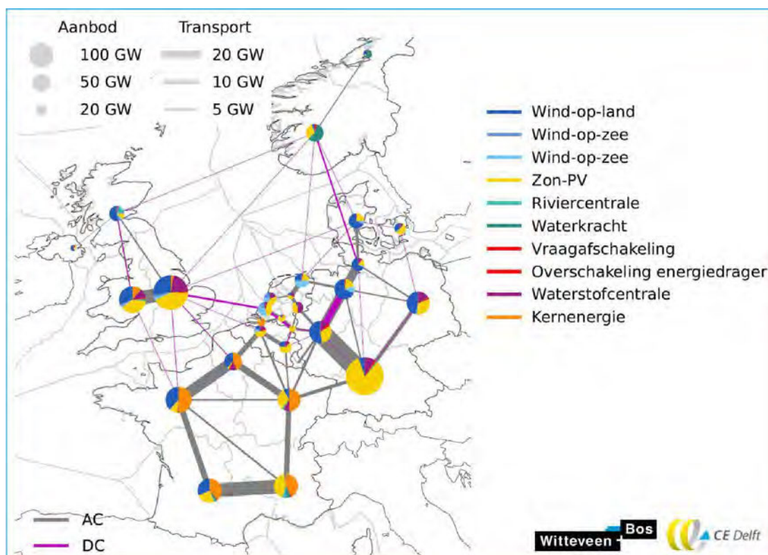
Figuur 5 - Systeemconfiguratie studie
