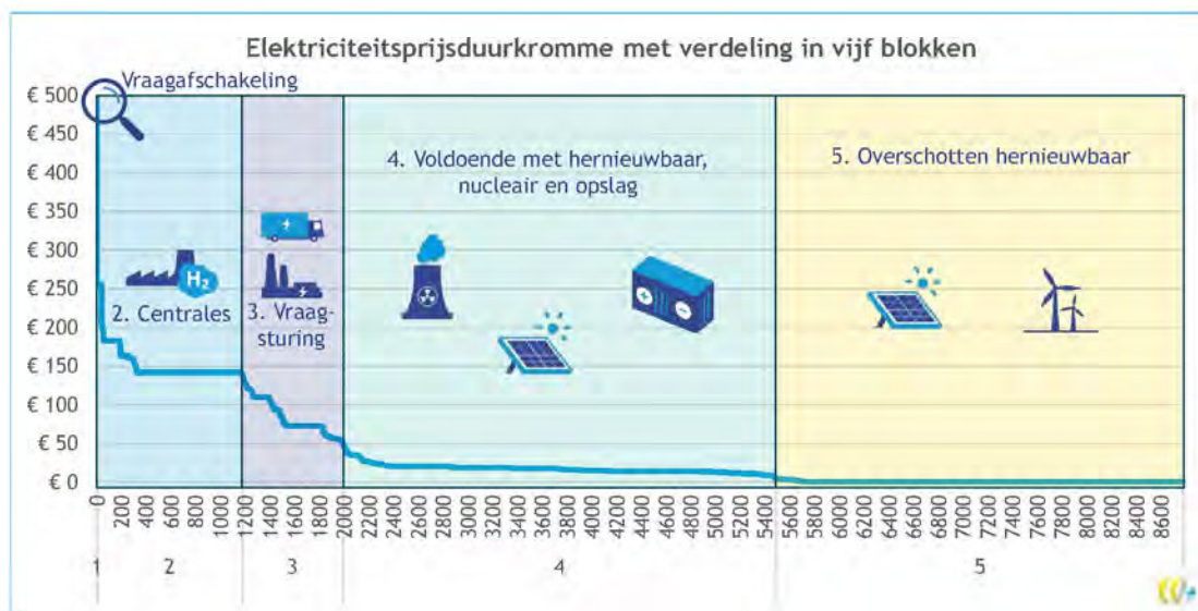
Figuur 2 - Elektriciteitsduurkromme 2035, referentiescenario
