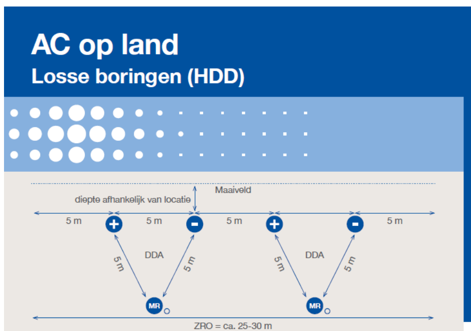
Figuur 3-17 Schematische weergave van een open ontgraving (boven) en boringen (onder) voor de wisselstroomkabels (AC) van Doordewind Alpha (DDA) en Beta (DDB)
