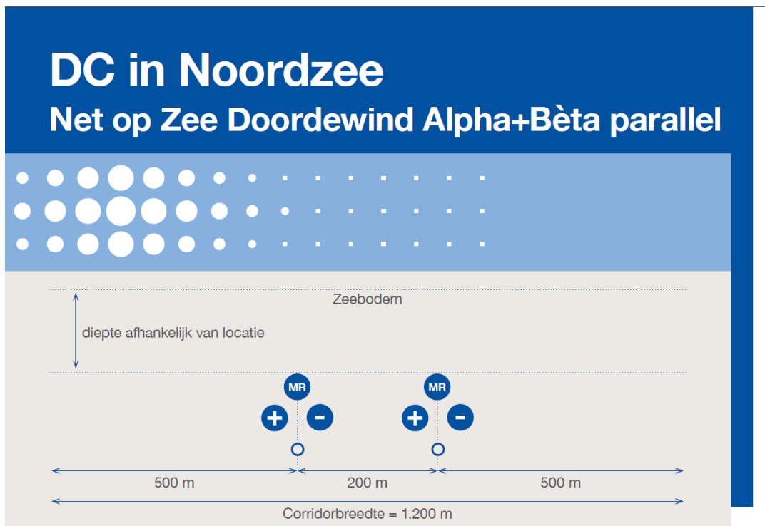
Figuur 3-6 Schematische weergave van de gelijkstroomkabels (DC) op zee
