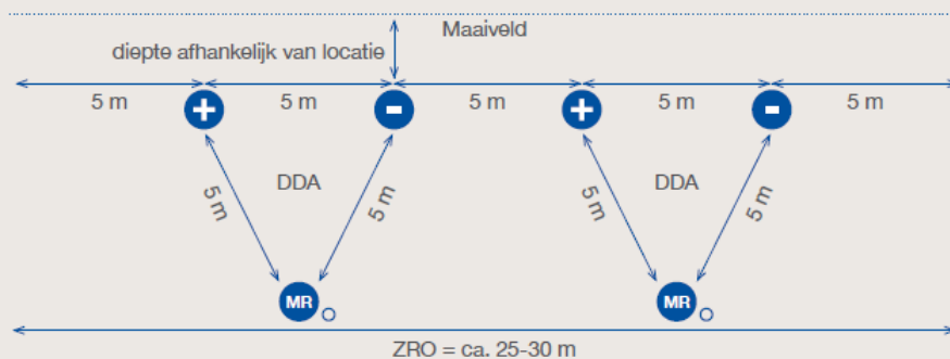
Figuur 3-12 Schematische weergave van een bundelboring (boven) of losse boringen (onder) voor de gelijkstroomkabels (DC) van Doordewind Alpha (DDA) en Beta (DDB)
