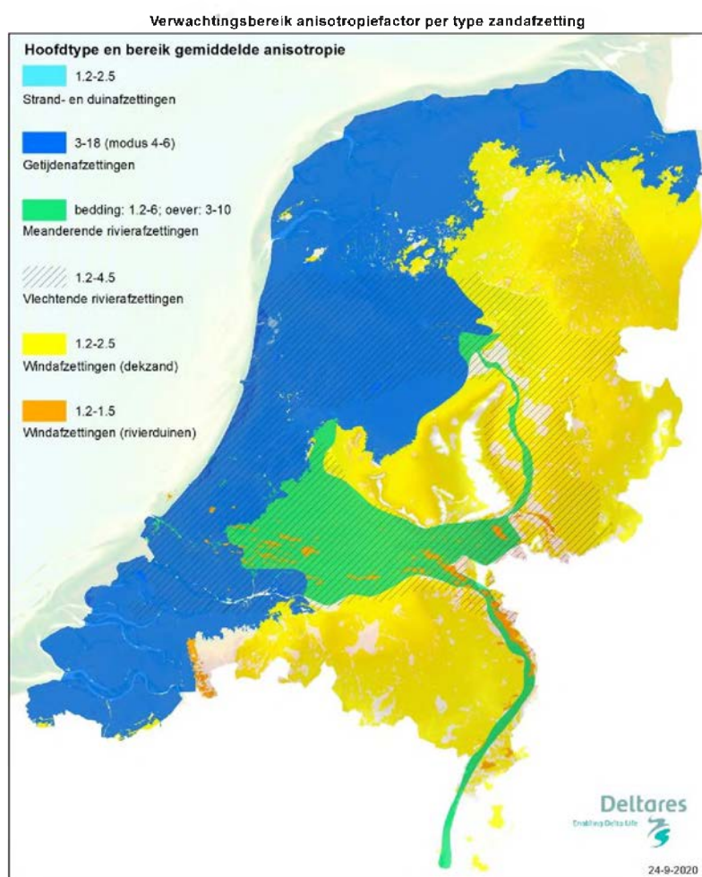
Figuur 2-2 Verwachte anisotropiefactor
