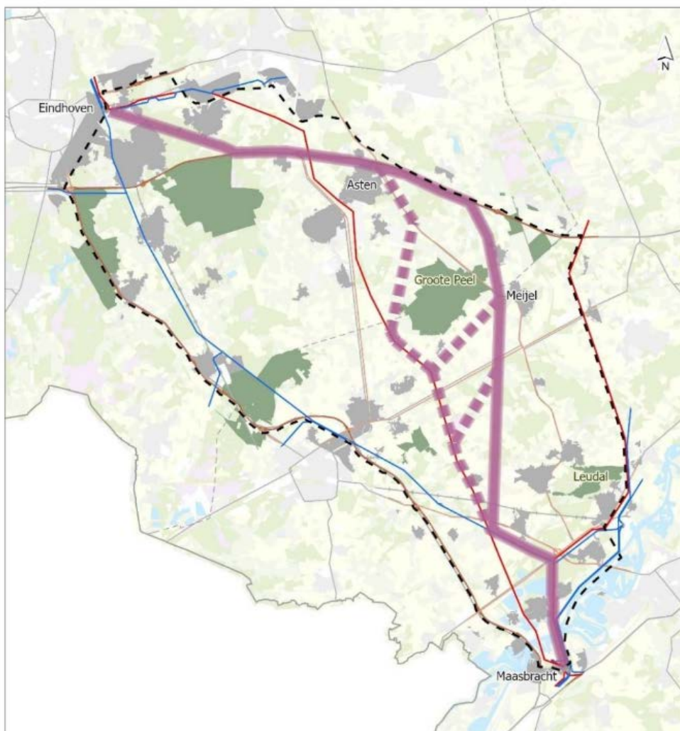
Afbeelding 17.4 Alternatief oost met varianten
