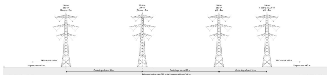
Figuur 6.30 Doorsnede van cumulatie van vier hoogspanningslijnen met bijbehorende belemmerende strook
