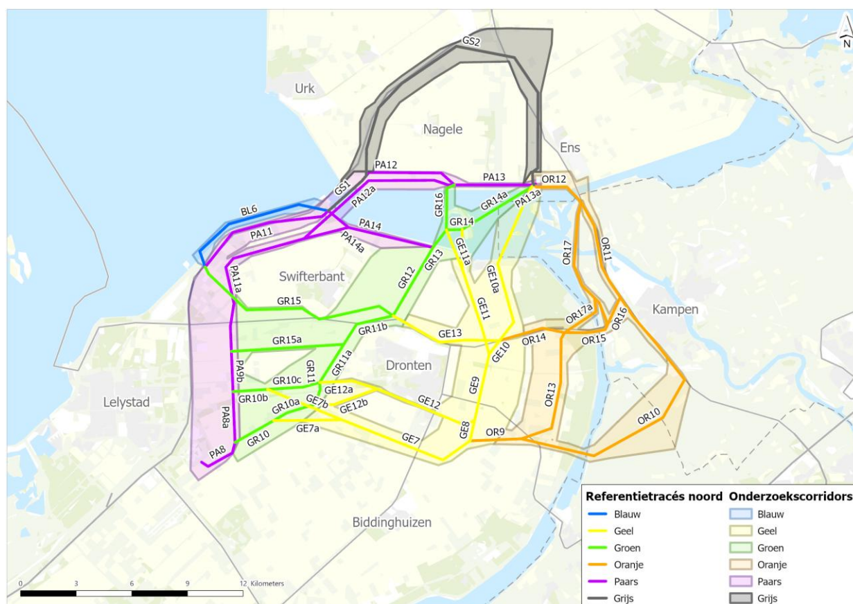
Figuur 1.8 Corridors met daarin de referentielijnen voor deelgebied noord
