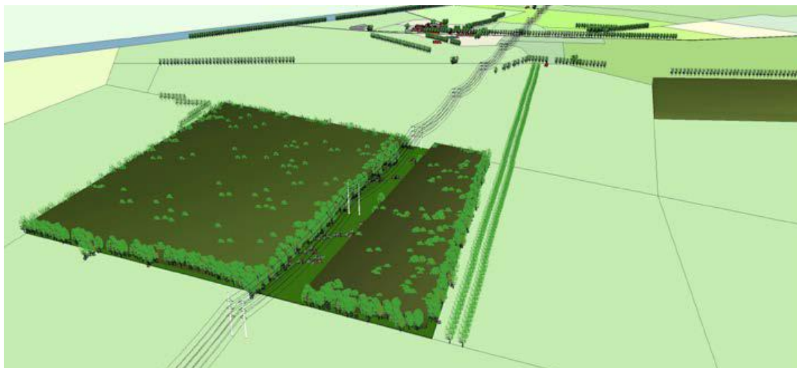
Figuur 8.6 Een bos wordt scherp doorsneden door een hoogspanningsverbinding (bron: landschap en hoogspanningsnet, 2017)
