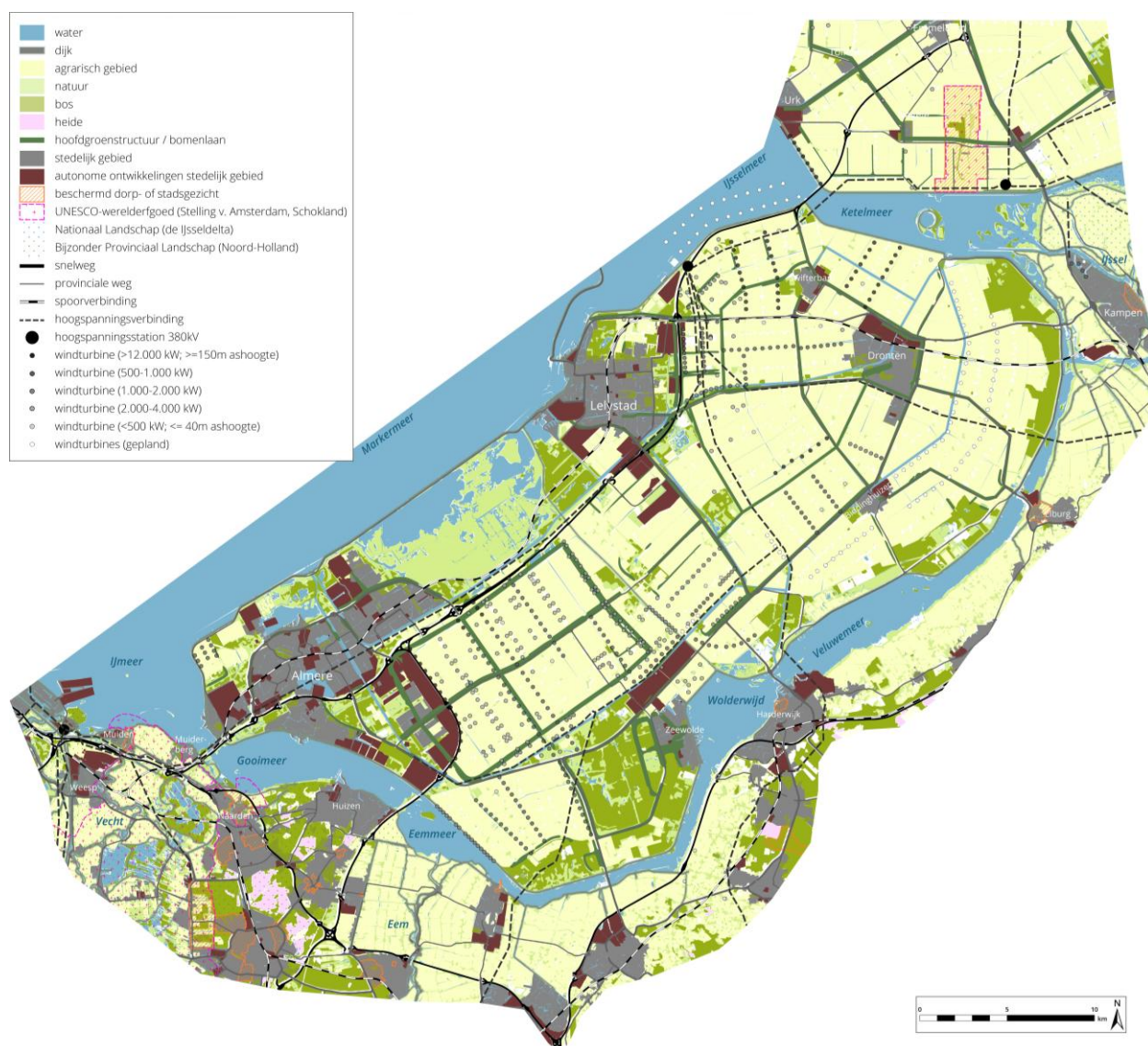
Figuur 4.3 Ruimtelijke analyse van het landschap binnen het onderzoeksgebied op lijnniveau
