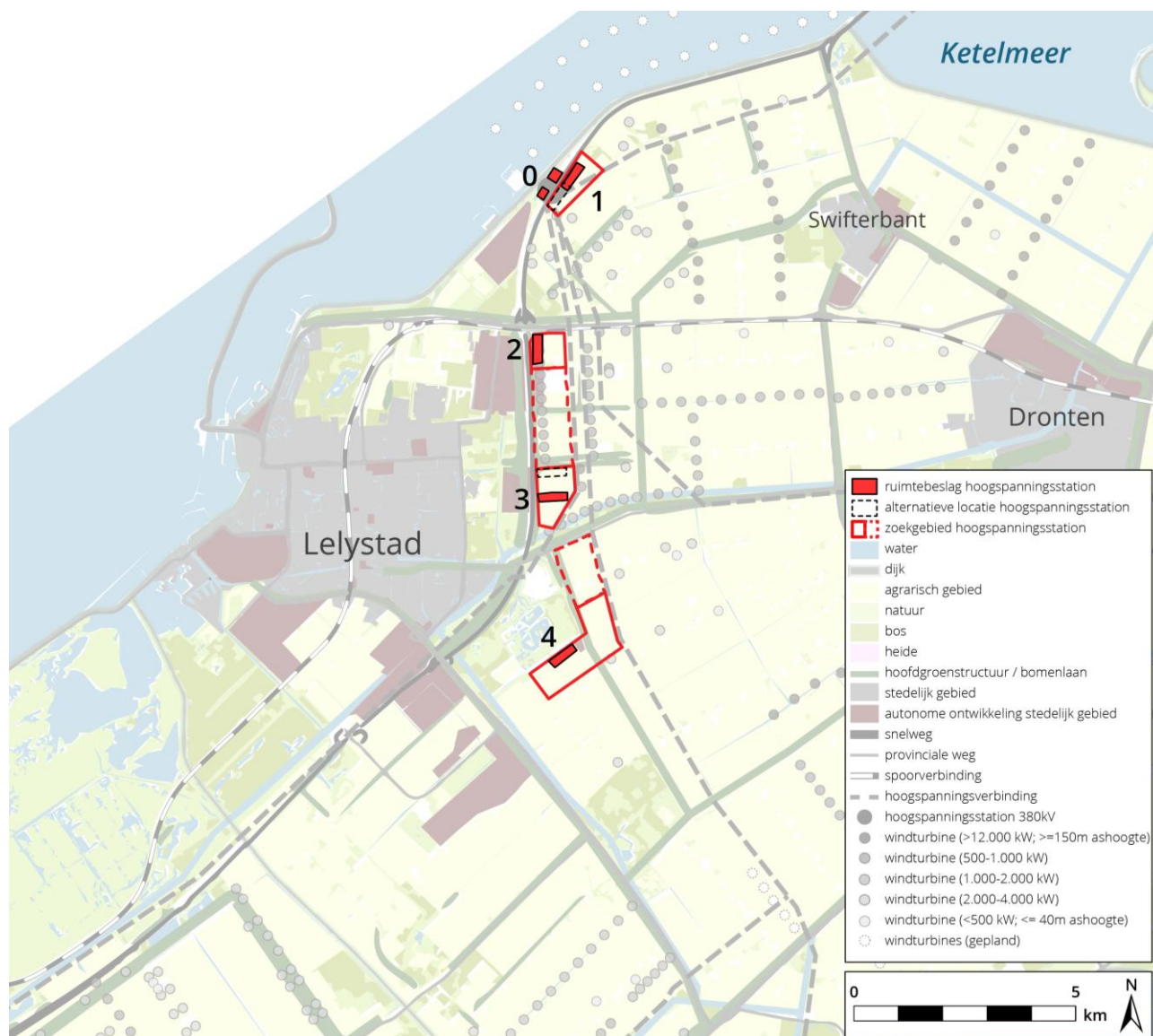
Figuur 8.2 Overzichtskaart locatiealternatieven Lelystad
