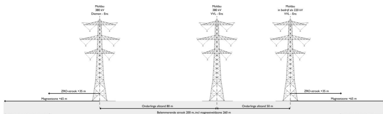
Figuur 6.29 Doorsnede van cumulatie van drie hoogspanningslijnen met bijbehorende belemmerende strook
