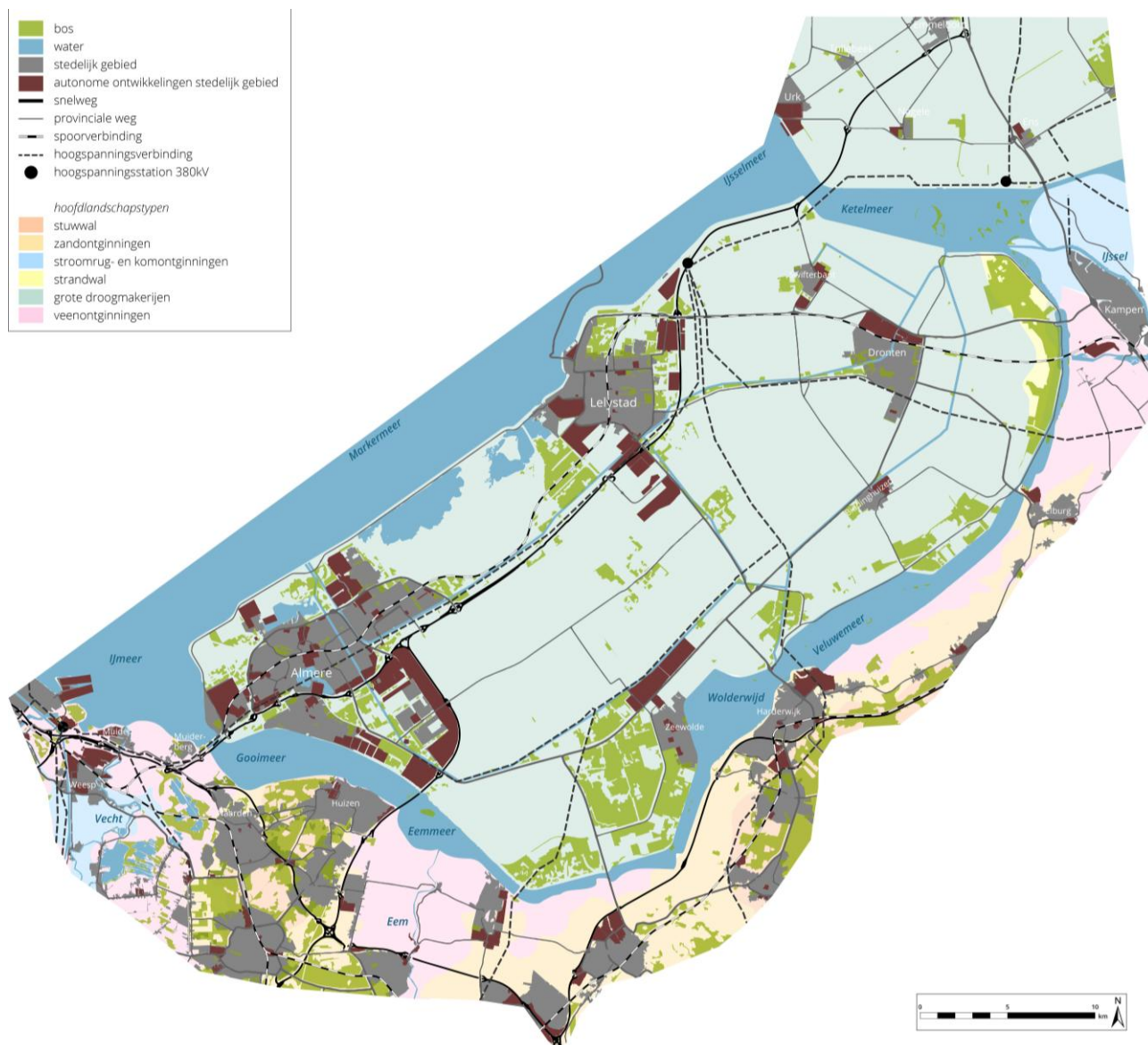
Figuur 4.2 Ruimtelijke analyse van het landschap binnen het onderzoeksgebied op tracéniveau
