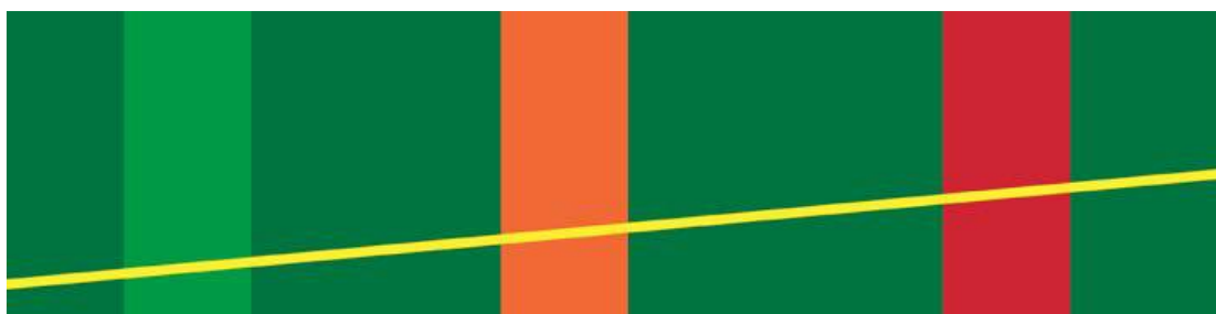
Figuur 3.2 Een autonome lijn in het landschap (bron: Landschap en hoogspanningsnet, 2017)
