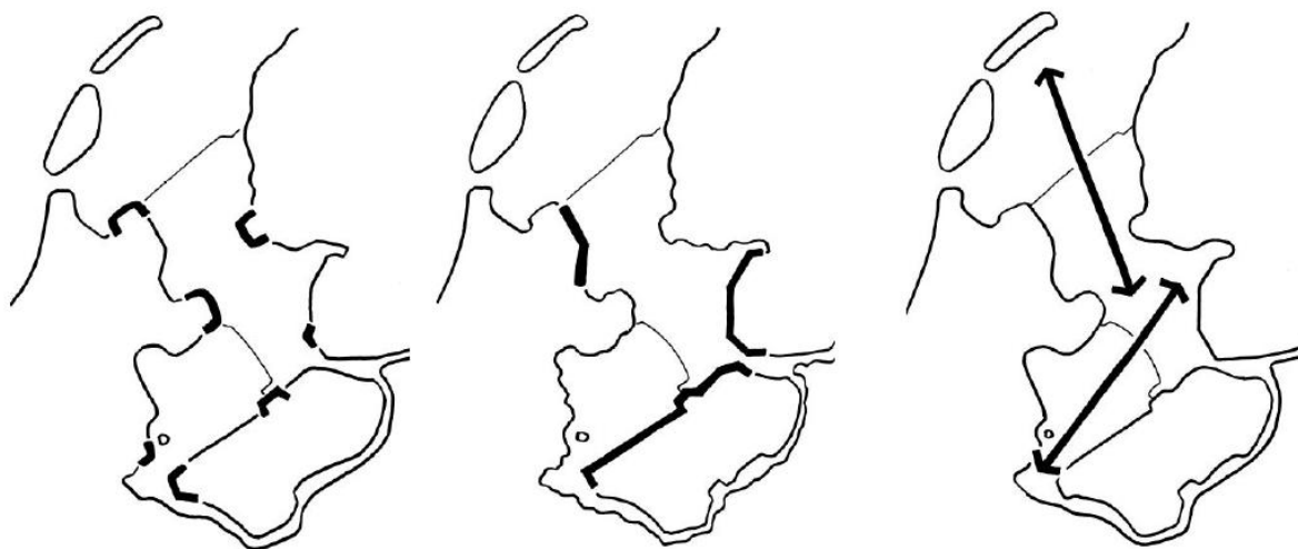
Figuur 4.15 (links) Opeenvolging van baaien en kapen (bron: Handreiking Omgevingskwaliteit IJsselmeergebied, 2020)
