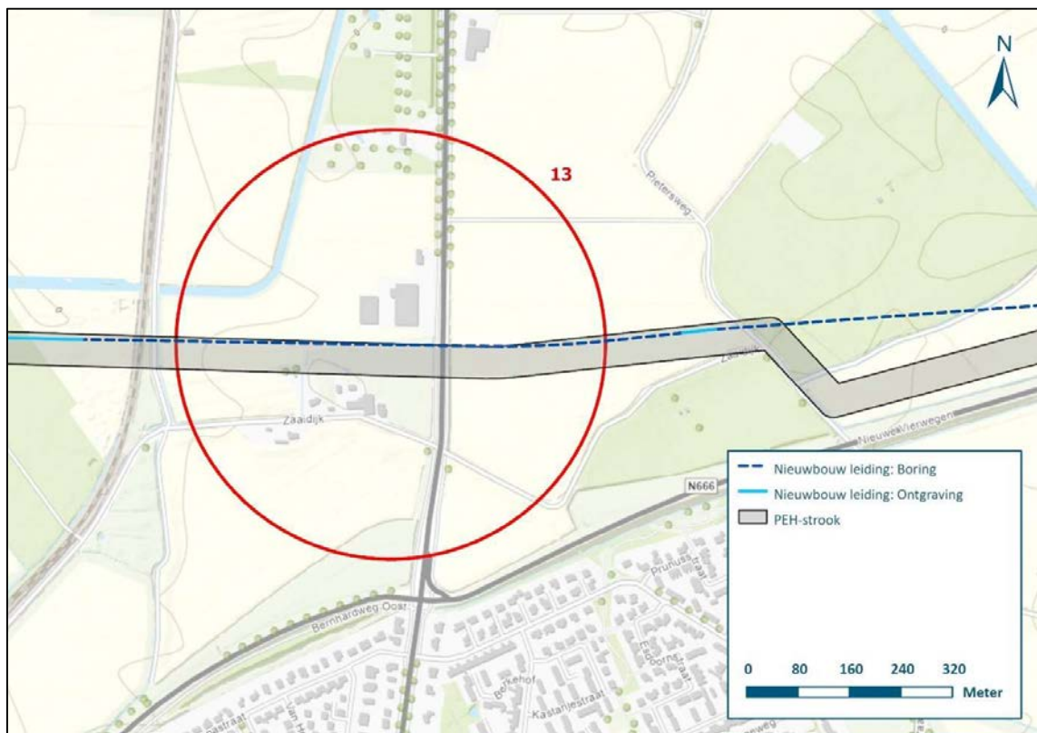
Figuur 15 | 13 Optimalisatie tracé Woensdrecht - Vlissingen
