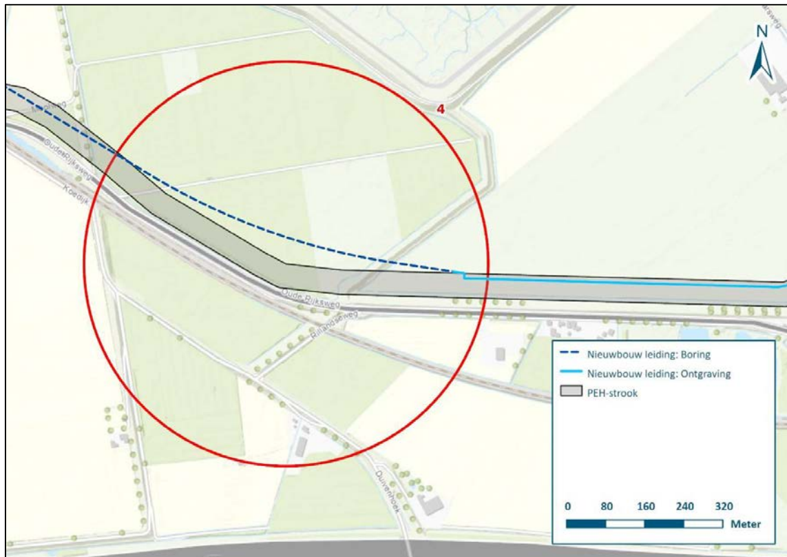
Figuur 6 | 04 Optimalisatie tracé Woensdrecht - Vlissingen
