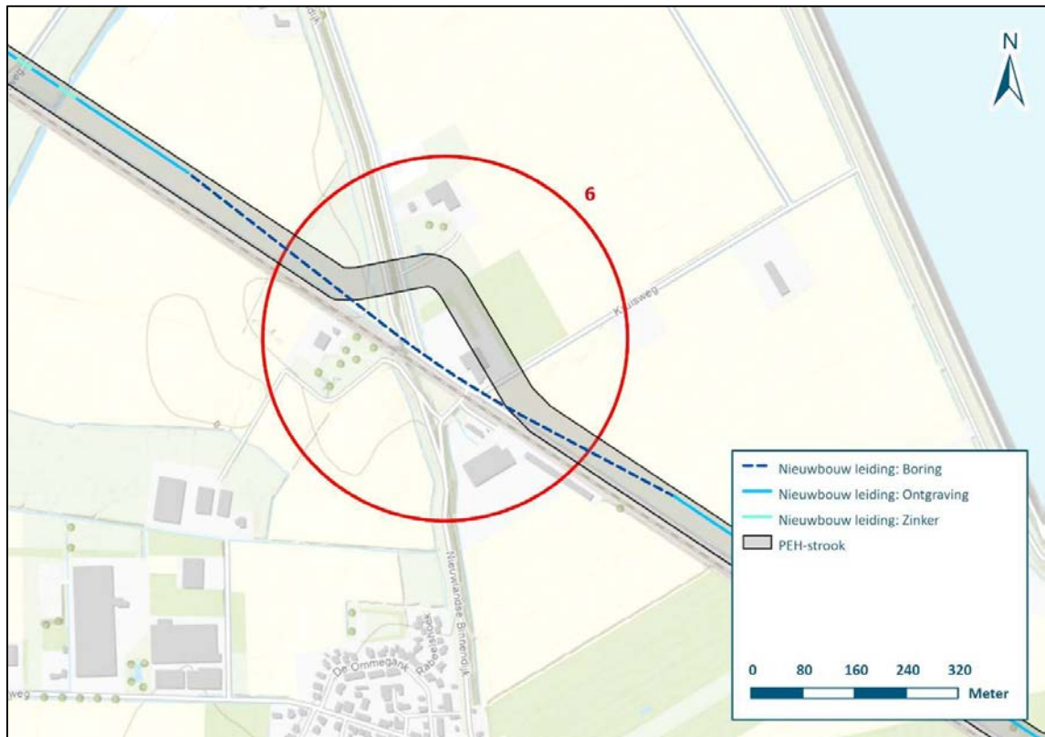
Figuur 8 | 06 Optimalisatie tracé Woensdrecht - Vlissingen
