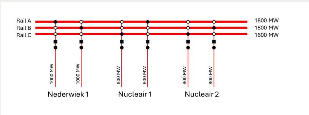
Figuur 11: Schematische weergave aansluitconfiguratie NW-1 en 3,2 GW nucleair NDLS380
