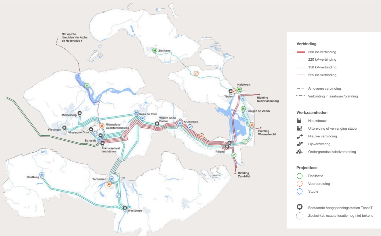
Figuur 5: Netkaart van het 380 kV-netwerk in Zeeland. Rode lijnen zijn 380 kV-circuits.
