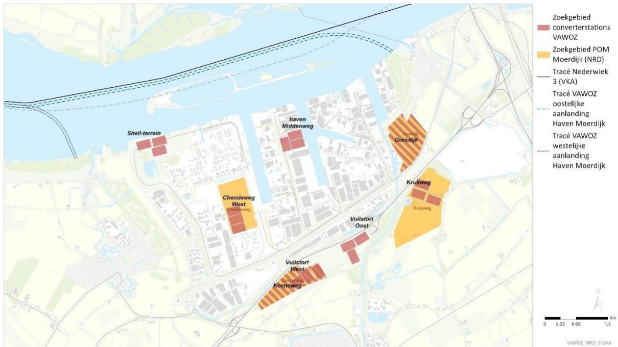
Figuur 2-17: Overzichtskartaal haven- en industrieterrein Moerdijk, met uittredepunt DC-kabelroute vanuit BWA aan de west- en oostkant van de haven.
