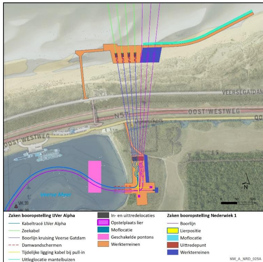
Figuur 2-2:- Overzichtskaart aanlanding met boringen twee parallelle Net op zee 2GW verbindingen IJmuiden Ver Alpha en Nederwiek 1 onder Veerse Gatdam
