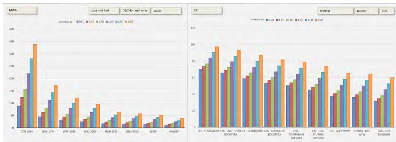
Figuur 2 Berekende warmtebehoefte woningen afhankelijk van vormfactor, ventilatiesysteem, bouwmassa (licht, zwaar) en isolatiegraad
