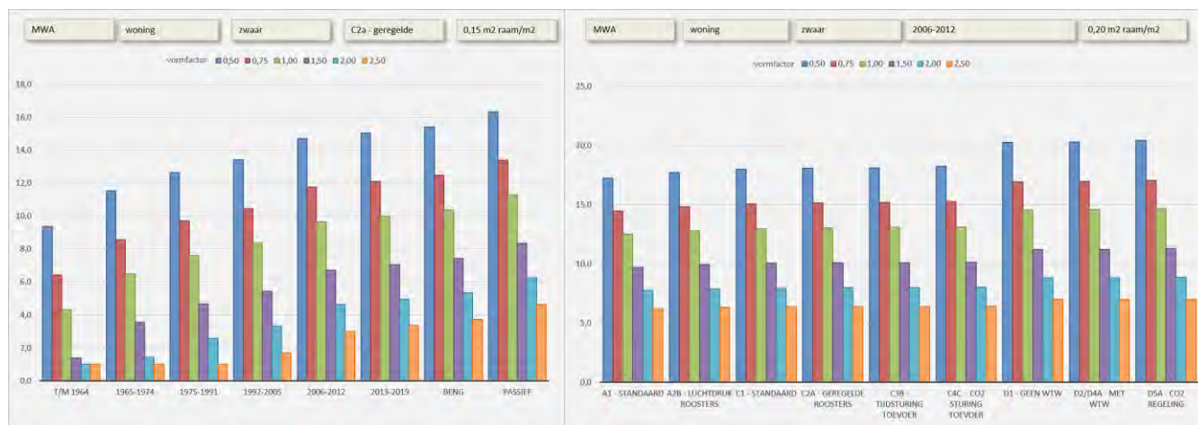
Figuur 3 Berekende koudebehoefte woningen afhankelijk van vormfactor, ventilatiesysteem, bouwmassa, raamoppervlak en isolatiegraad
